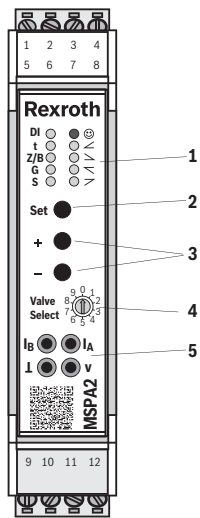
Abb. 5: Frontansicht mit Bedien- und Anzeigeelementen
