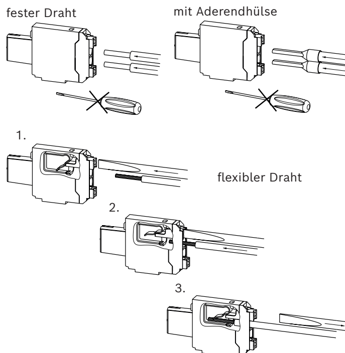
Abb. 3: XG20/XG21: „PUSH-IN“-Kontakt
