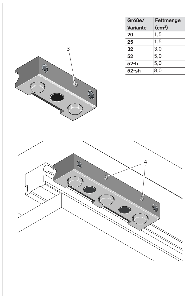
Fig. 93: Wartung Kassetten
