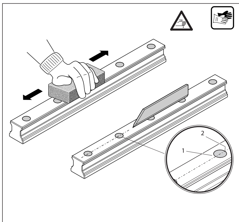
Fig. 25: Montage Abdeckkappen aus Stahl abschließen
