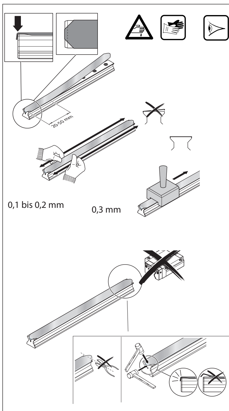
Fig. 37: Montage Abdeckbänder bei passender Abdeckbandlänge
