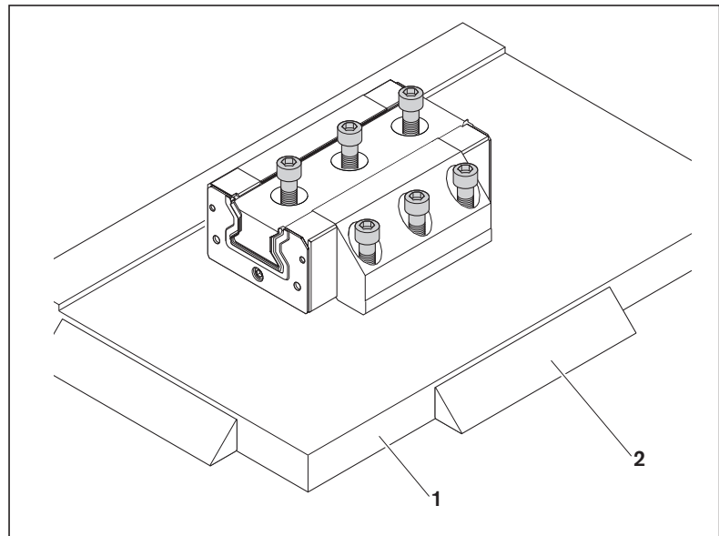
Fig. 63: Schwerlast-Rollenwagen vormontieren
