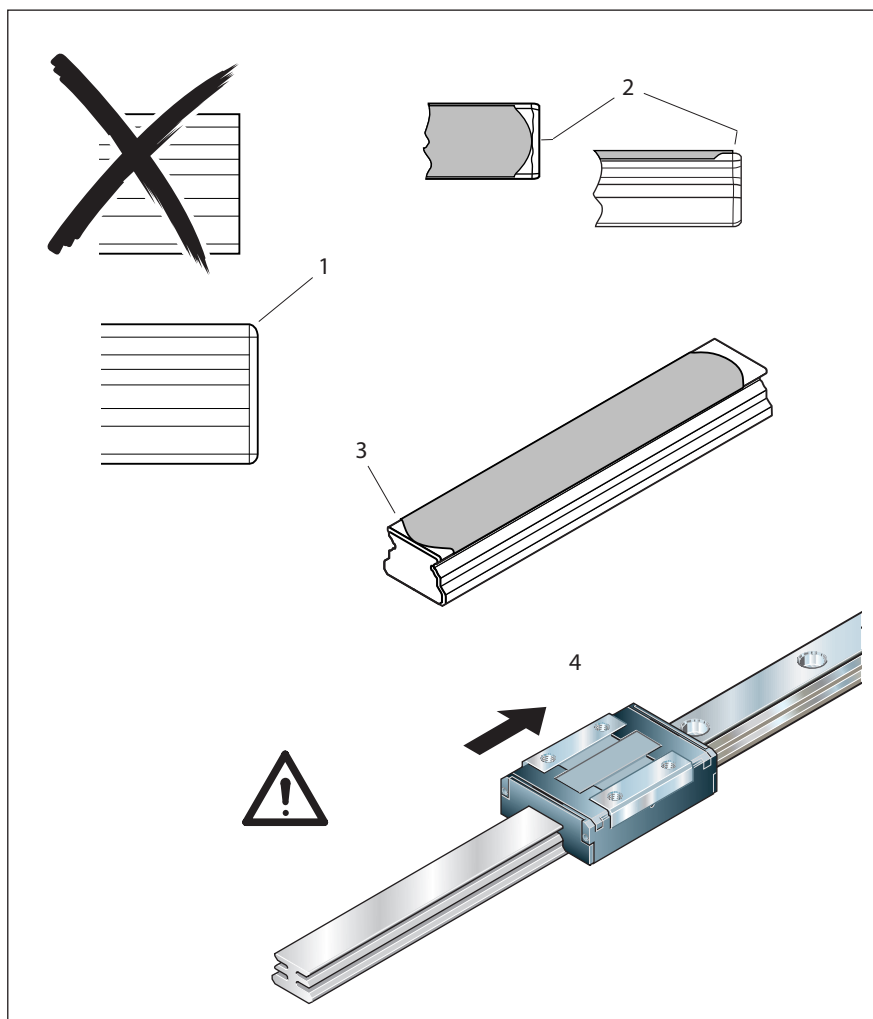
Fig. 67: Führungswagen MKS aufschieben
