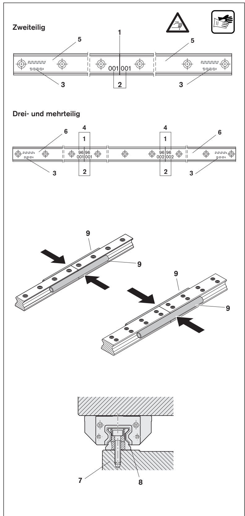
Fig. 8: Mehrteilige Führungsschienen bereitlegen
