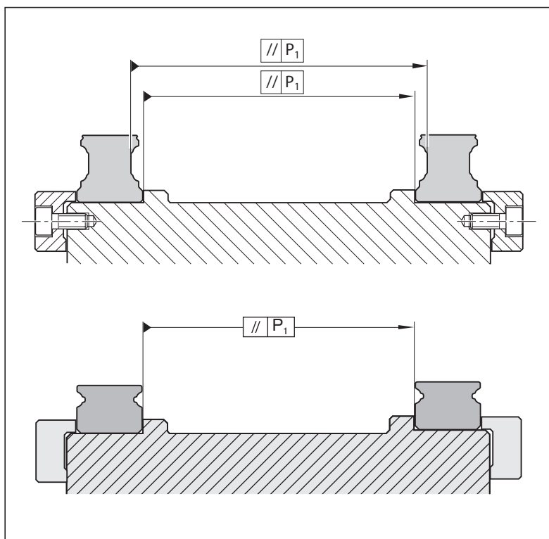
Fig. 16: Parallelität der Führungsschienen prüfen
