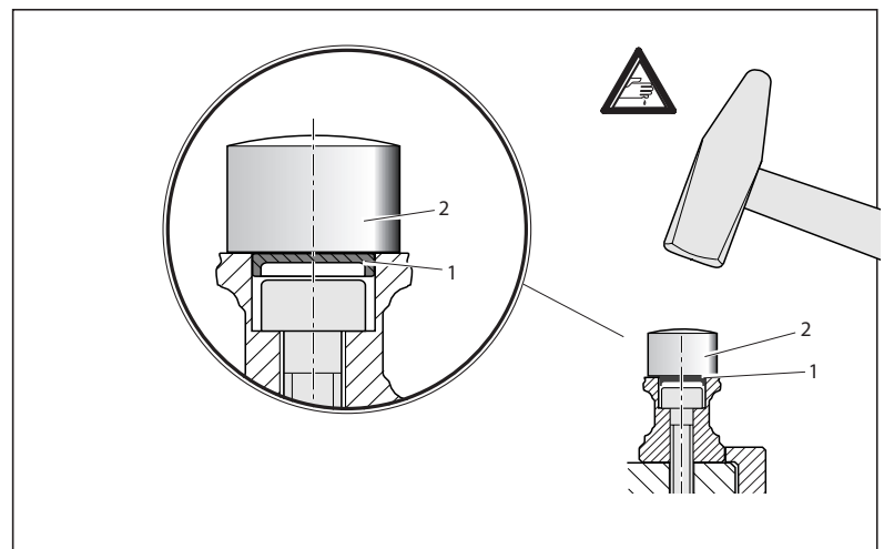
Fig. 21: Abdeckkappen aus Kunststoff montieren
