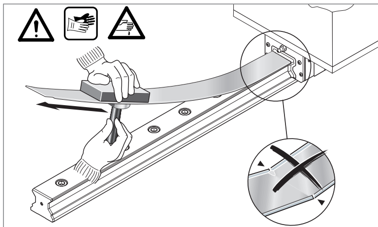
Fig. 42: Abdeckband aufweiten
