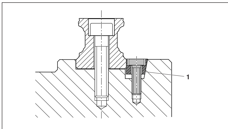
Fig. 15: Keilleisten montieren
