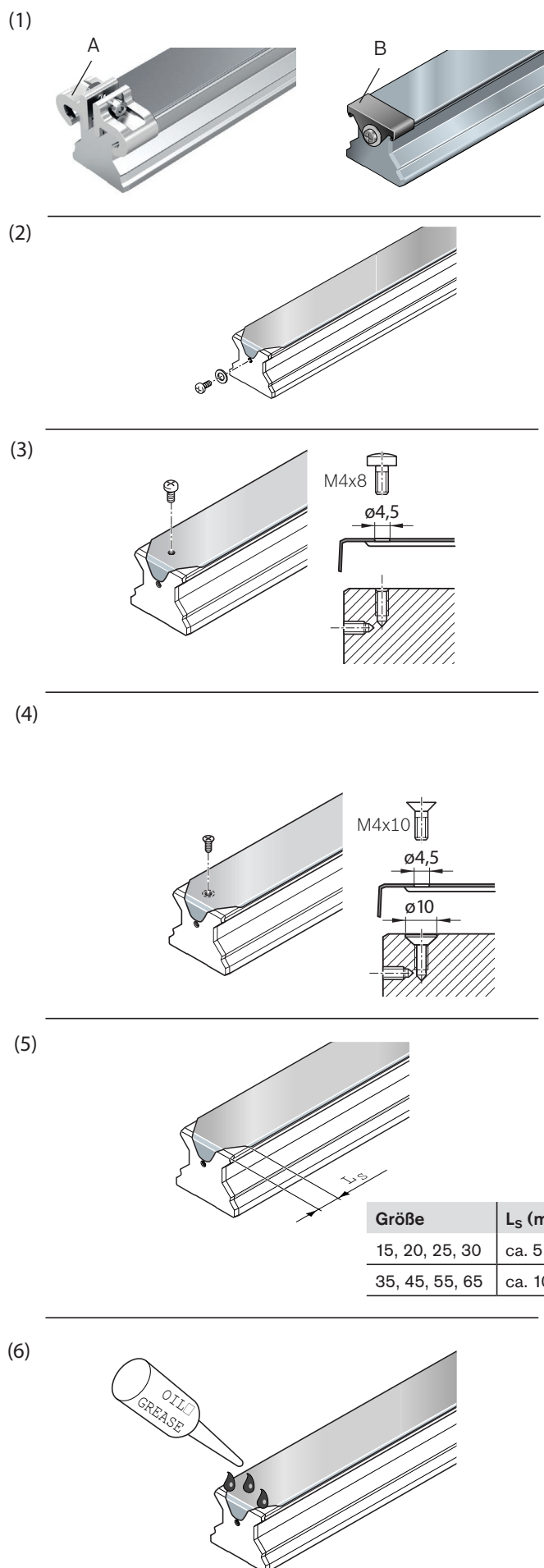
Fig. 51: Abdeckband sichern
