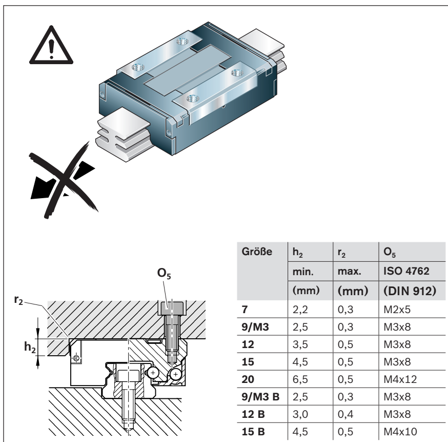
Fig. 66: Montage MKS vorbereiten
