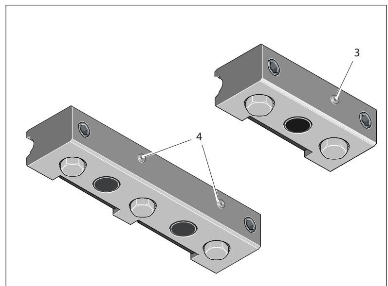
Fig. 91: Kassetten in Betrieb nehmen
