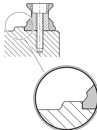
Fig. 11: Führungsschienen vorbereiten
