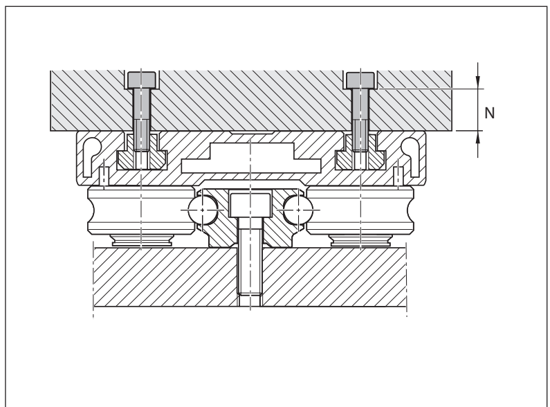
Fig. 82: Geführtes Bauteil auf Profilführungswagen montieren
