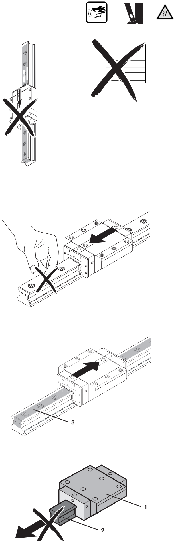
Fig. 52: Montage Führungswagen (Hinweise)
