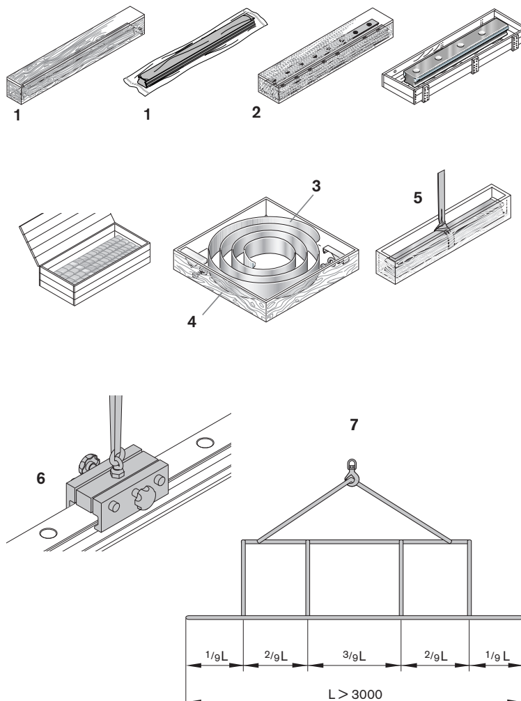
Fig. 4: Gewicht und Lieferung Führungsschienen
