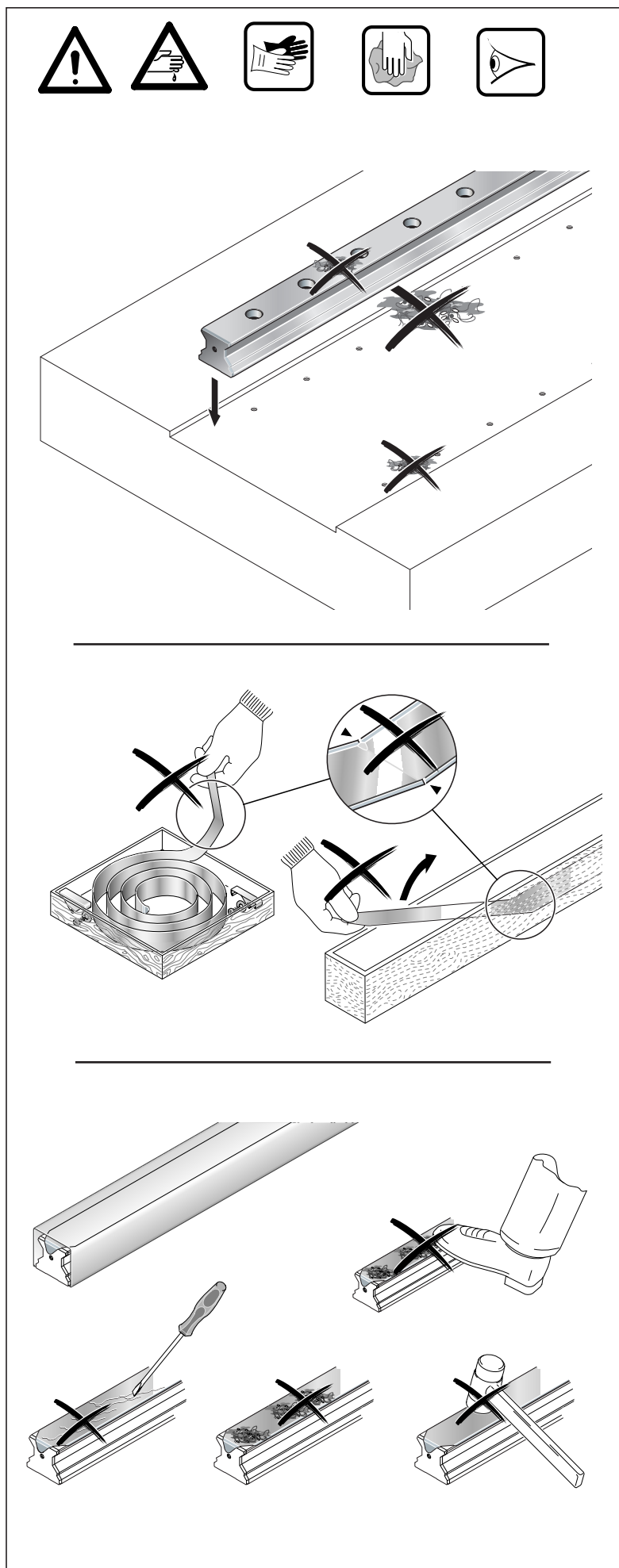
Fig. 33: Montagegrundlagen Abdeckband
