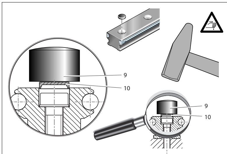
Fig. 78: Kunststoffabdeckkappen montieren
