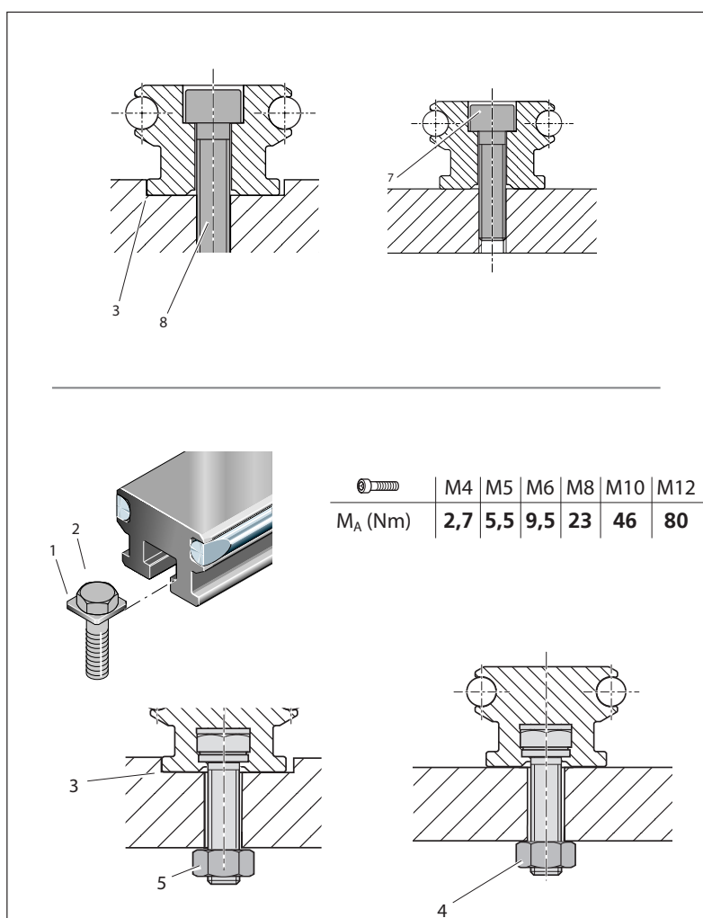
Fig. 76: LRF FS/FS mit Nut montieren
