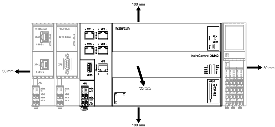
Abb. 10-2: Mindestabstände für die Zirkulation der Umgebungsluft
