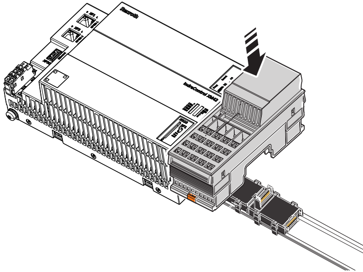
Abb. 10-9: S20-Module aufsetzen
