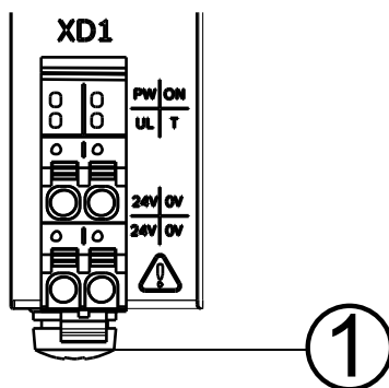
Abb. 10-16: Position der Erdungsschraube
