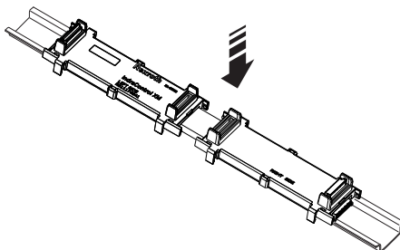
Abb. 10-6: Steuerungsbussockel
