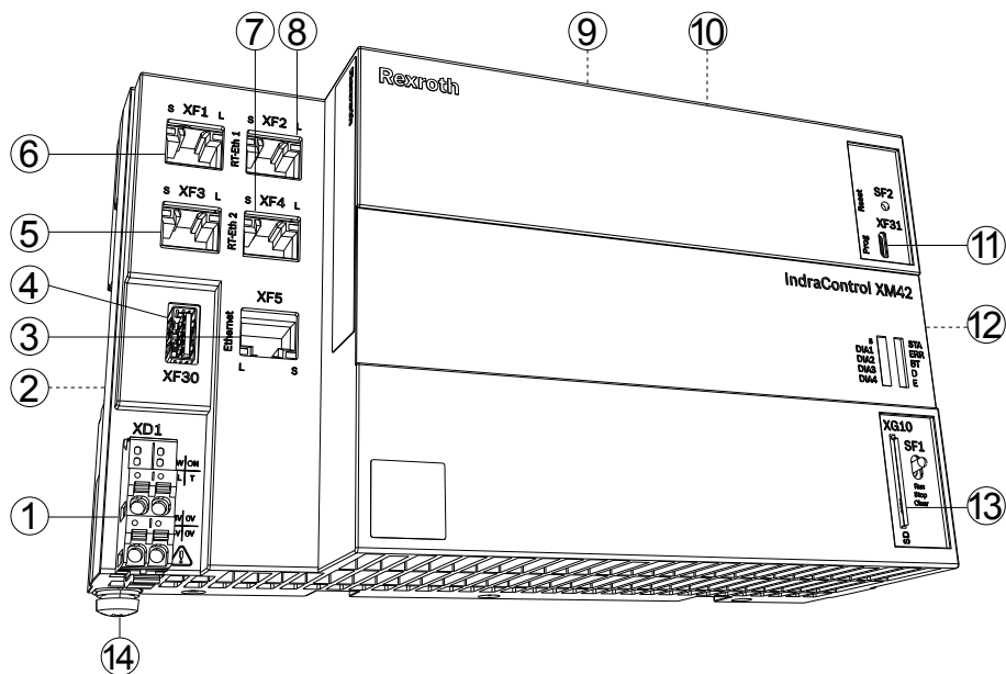
Abb. 9-1: Schnittstellen
