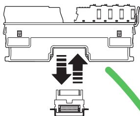
Abb. 10-5: Module nur senkrecht aufsetzen und abnehmen
