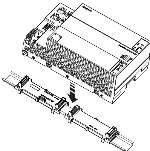
Abb. 10-7: Steuerung aufrasten
