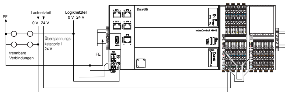
Abb. 10-15: Aufbau mit zwei Netzteilen
