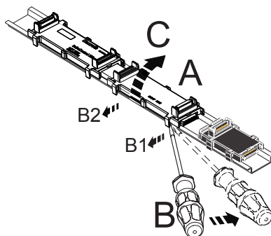
Abb. 10-12: Steuerbussockel von der Hutschiene nehmen
