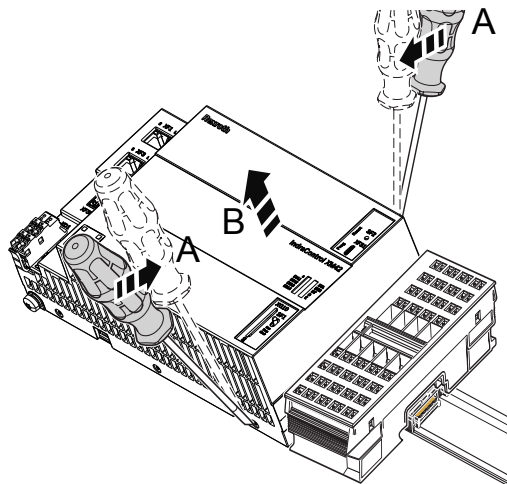
Abb. 10-11: Steuerung von der Hutschiene nehmen
