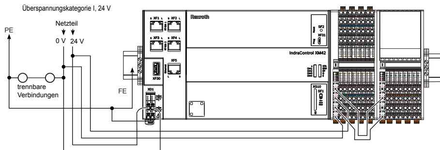
Abb. 10-14: Aufbau mit einem Netzteil
