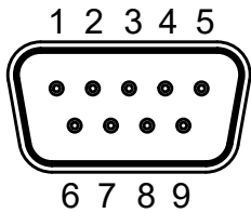
Abb. 9-12: Pinbelegung RS-232, 9-polig, männlich
