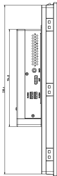
Abb. 10-11: Gehäusemaße Gerät VR3121, linke Seitenansicht
