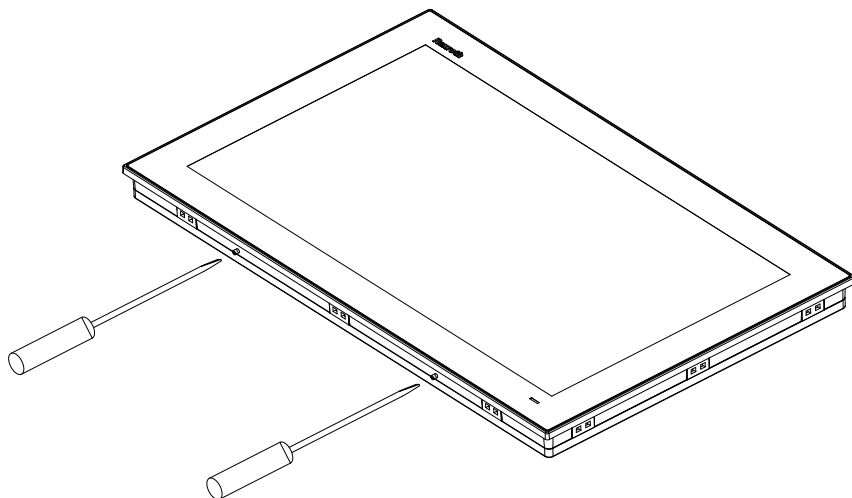
Abb. 10-15: Montageschrauben an der Unterseite des Display
