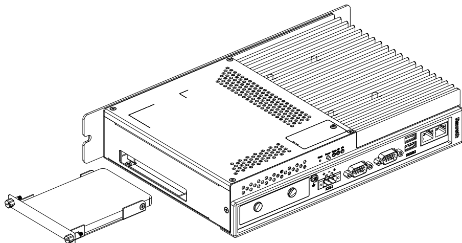
Abb. 10-13: Massenspeichereinbau
