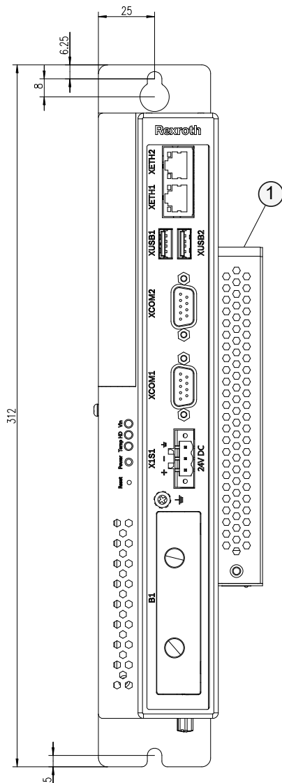
Abb. 10-1: Montagemaße für Gerät, Buchmontage
