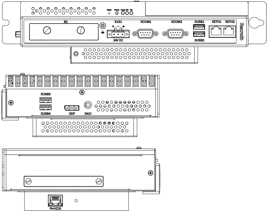
Abb. 9-2: Schnittstellen PR31 mit CDI+-Schnittstelle. An der Frontseite (oben), an der oberen Gehäuseseite (mitte) dem Massenspeicher-Einschub und der CDI+-Schnittstelle an der Gehäuseunterseite (unten).
