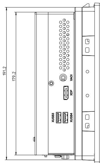
Abb. 10-5: Gehäusemaße Gerät VR3110, linke Seitenansicht
