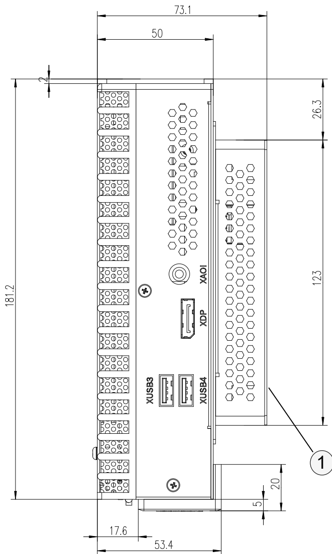
Abb. 10-3: Gehäusemaße, Ansicht von oben
