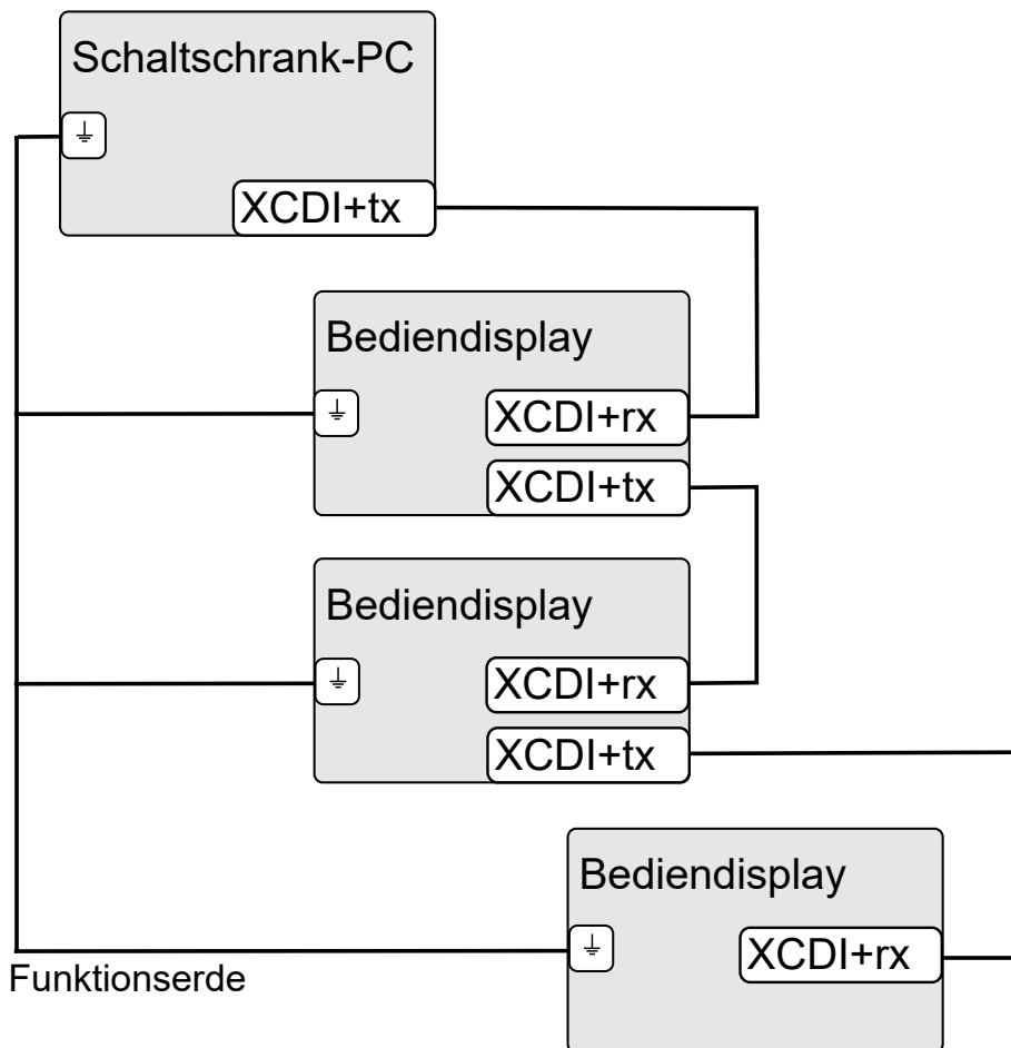
Abb. 10-22: Verdrahtung von bis zu drei Bediendisplays mittels CDI+ an einem Schaltschrank-PC
