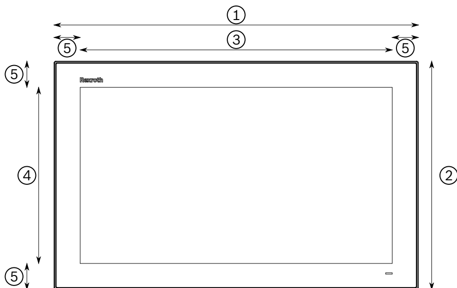
Abb. 10-4: Frontansicht Panel-PC
