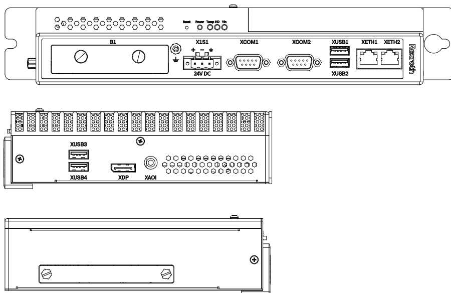
Abb. 9-1: Schnittstellen PR31 ohne CDI+-Schnittstelle. An der Frontseite (oben), an der oberen Gehäusesseite (mitte) und dem Massenspeicher-Einschub an der Gehäuseunterseite (unten).
