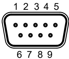
Abb. 9-10: Pinbelegung RS-422/485, 9-polig, männlich
