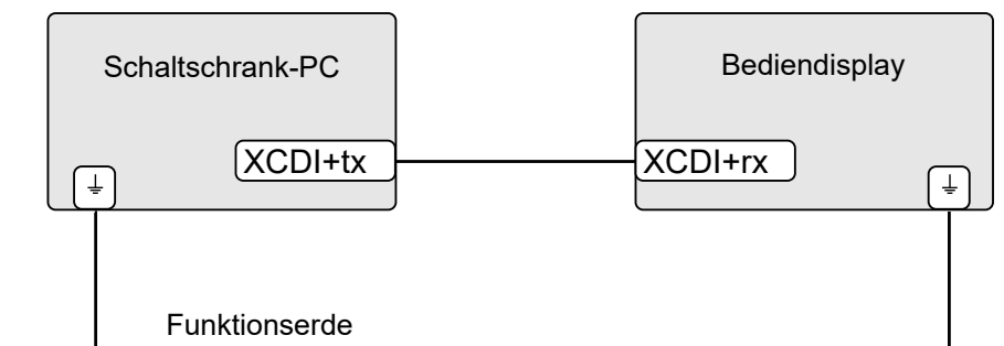
Abb. 10-21: Verdrahtung des Schaltschrank-PCs mit einem Bediendisplay
