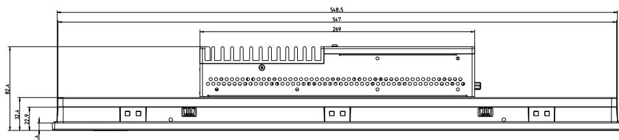
Abb. 10-12: Gehäusemaße Gerät VR3121, Ansicht von oben
