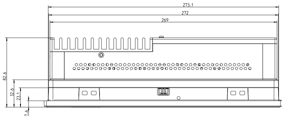
Abb. 10-6: Gehäusemaße Gerät VR3110, Ansicht von oben
