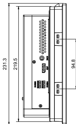
Abb. 10-7: Gehäusemaße Gerät VR3112, linke Seitenansicht
