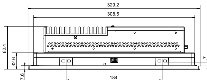
Abb. 10-8: Gehäusemaße Gerät VR3112, Ansicht von oben
