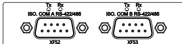
Abb. 9-9: Optionales Erweiterungsmodul RS-422/485, galvanisch getrennt
