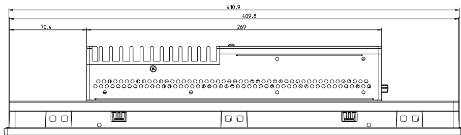
Abb. 10-10: Gehäusemaße Gerät VR3115, Ansicht von oben
