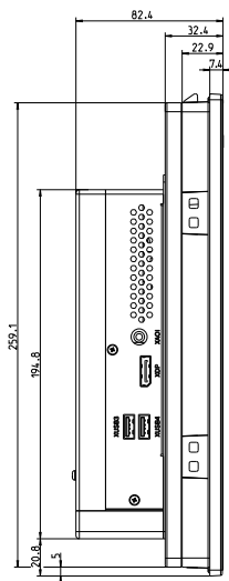
Abb. 10-9: Gehäusemaße Gerät VR3115, linke Seitenansicht
