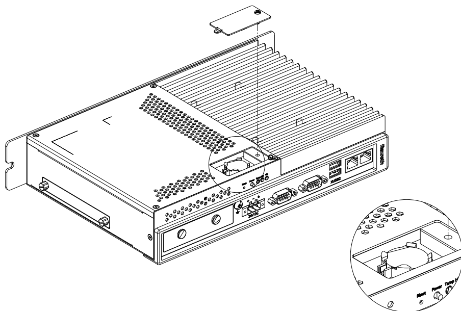
Abb. 10-14: CMOS-Batterie austauschen
