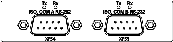
Рис. 9-11: Опциональный модуль расширения RS-232 с гальванической развязкой
