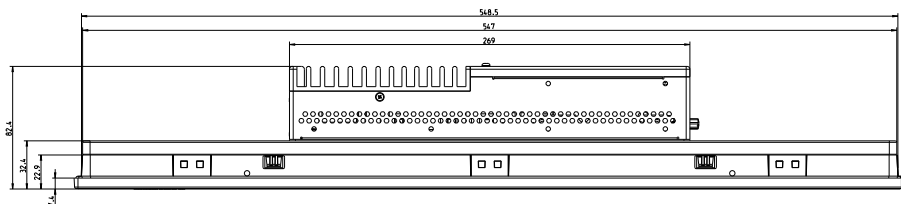
Рис. 10-12: Размеры корпуса устройства VR3121, вид сверху
