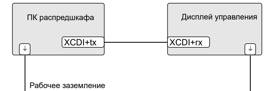
Рис. 10-21: Проводное соединение ПК для распределительных шкафов с дисплеем управления
