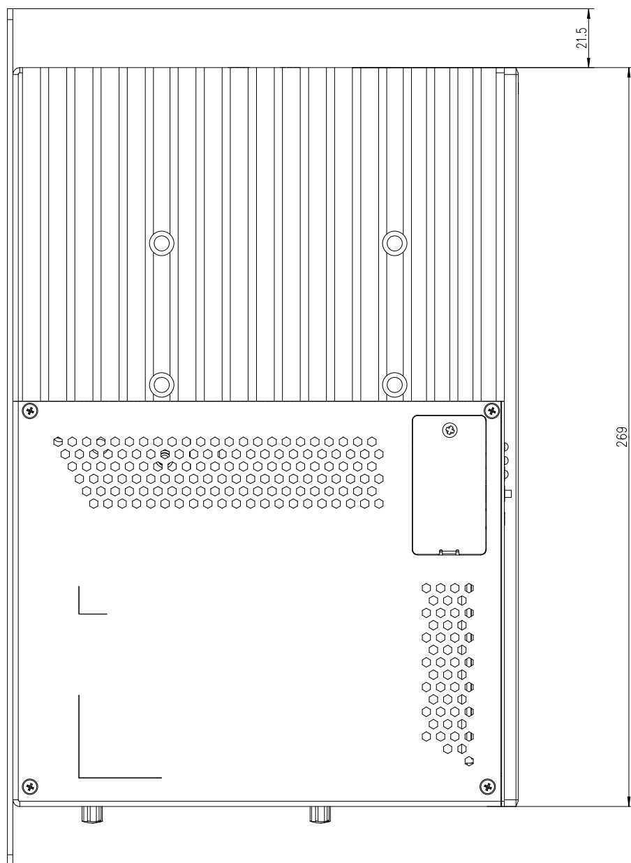
Рис. 10-2: Размеры корпуса, вид слева
