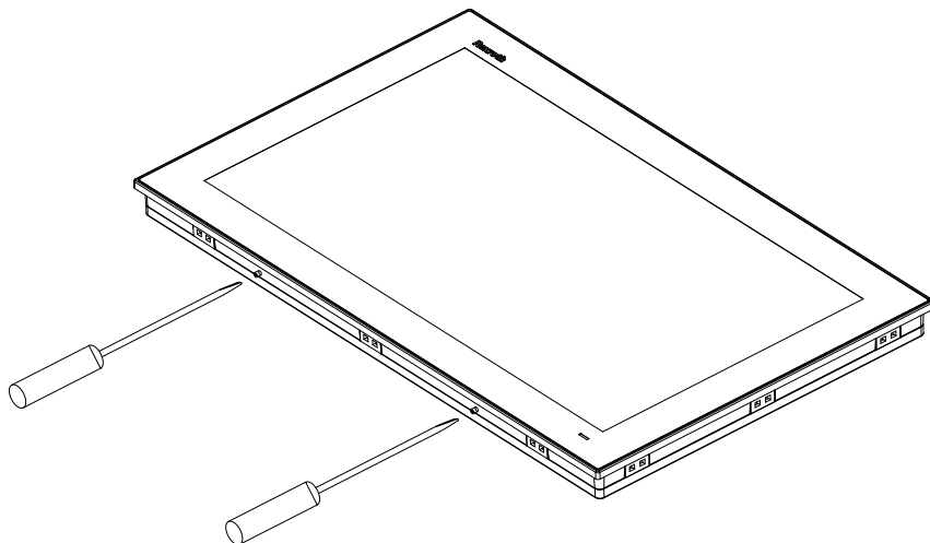
Рис. 10-15: Монтажные винты на нижней стороне дисплея
