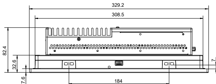
Рис. 10-8: Размеры корпуса устройства VR3112, вид сверху
