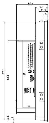
Рис. 10-9: Размеры корпуса устройства VR3115, вид слева
