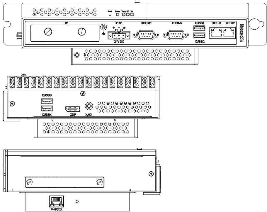
Рис. 9-2: Подключения PR31 с интерфейсом CDI+. На передней стороне (вверху), на верхней стороне корпуса (в середине) и ячейка для накопителя данных и гнездо интерфейса CDI+ на нижней стороне корпуса (внизу).
