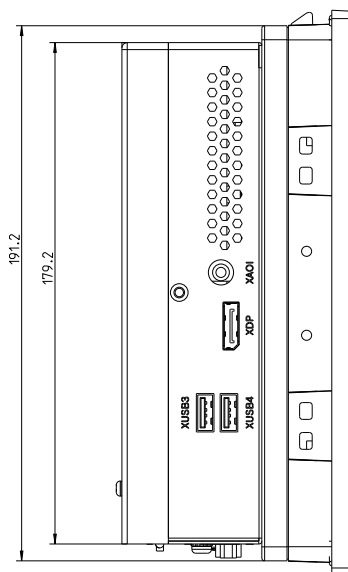
Рис. 10-5: Размеры корпуса устройства VR3110, вид слева
