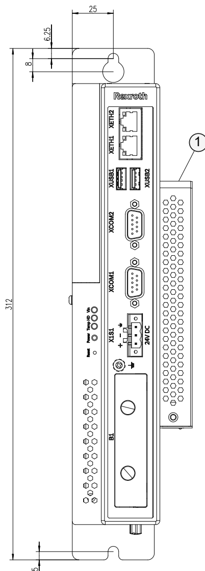
Рис. 10-1: Монтажные размеры устройства, «книжный» монтаж
