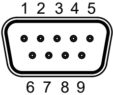
Рис. 9-10: Раскладка контактов RS-422/485, 9-полюсный штекер
