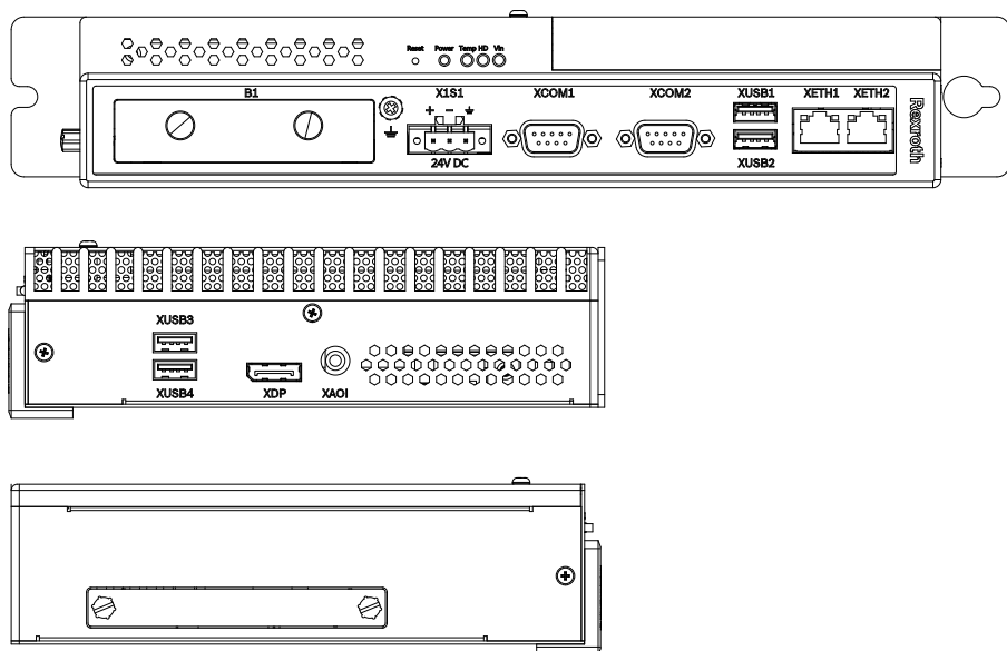
Рис. 9-1: Подключения PR31 без интерфейса CDI+. На передней стороне (вверху), на верхней стороне корпуса (в середине) и ячейка для накопителя данных на нижней стороне корпуса (внизу).
