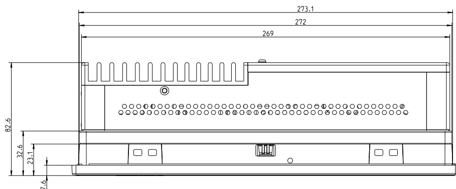
Рис. 10-6: Размеры корпуса устройства VR3110, вид сверху
