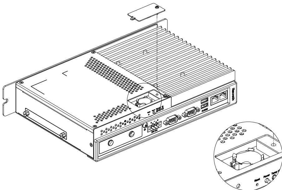
Рис. 10-14: Замена CMOS-батареи
