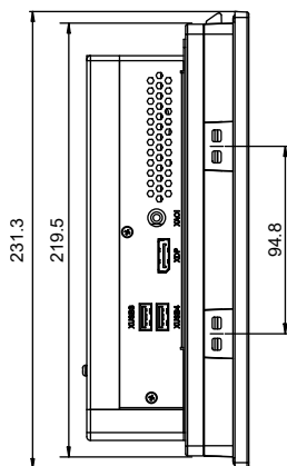
Рис. 10-7: Размеры корпуса устройства VR3112, вид слева
