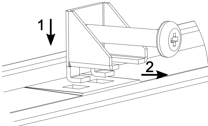
Рис. 10-18: Установка крепежного элемента в отверстие
