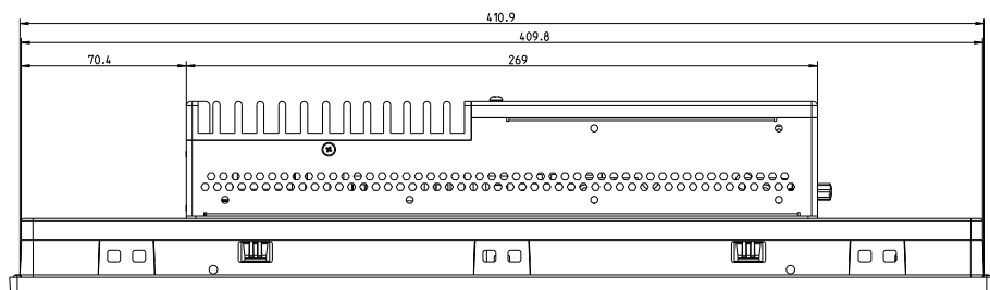
Рис. 10-10: Размеры корпуса устройства VR3115, вид сверху
