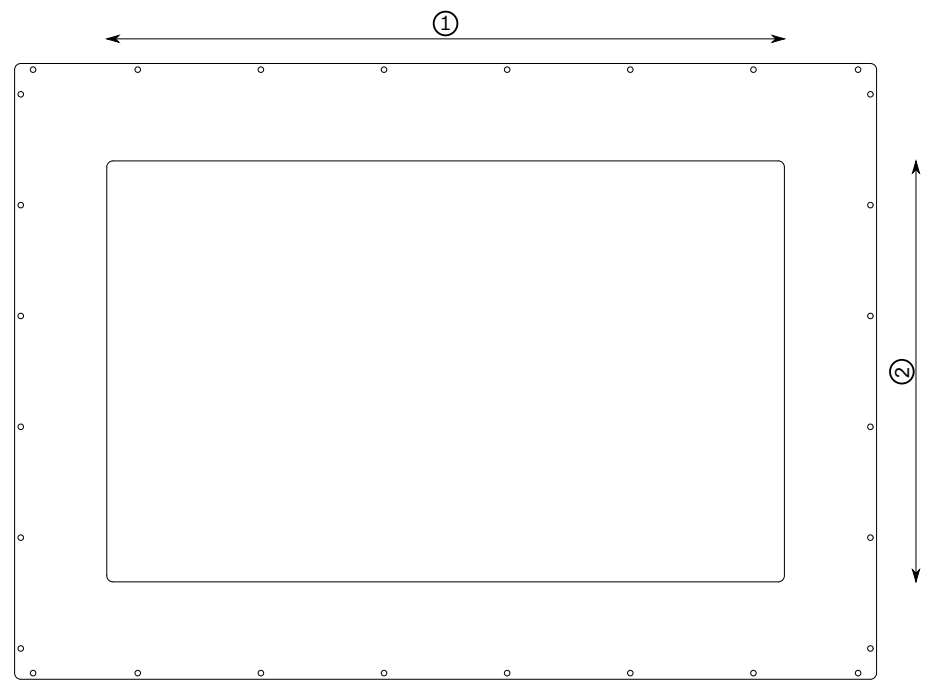
Рис. 10-20: Монтажный вырез
