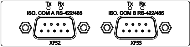
Рис. 9-9: Опциональный модуль расширения RS-422/485 с гальванической развязкой
