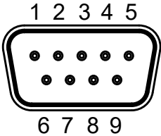
Рис. 9-12: Раскладка контактов RS-232, 9-полюсный штекер
