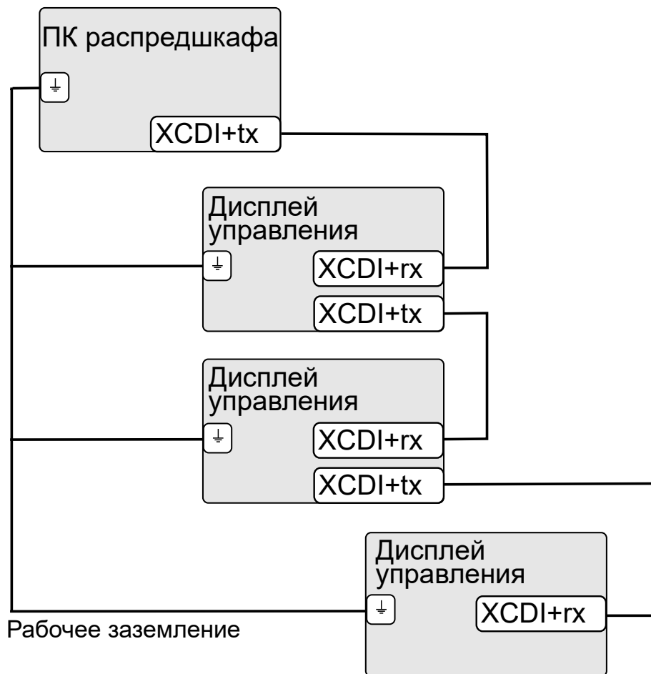
Рис. 10-22: Подключение до трех дисплеев управления к одному ПК для распределительных шкафов с помощью интерфейса CDI+
