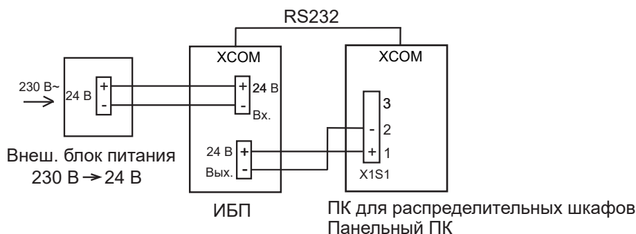
Рис. 10-23: Общая схема подключения — блок питания, ИБП и ПК для распределительных шкафов
