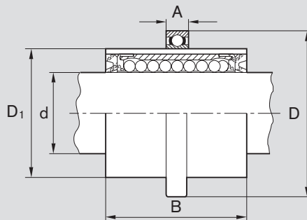
Avec roulement à billes à gorge profonde, série 618
