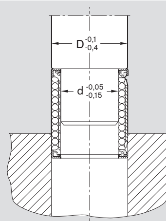
Mandrin de montage
