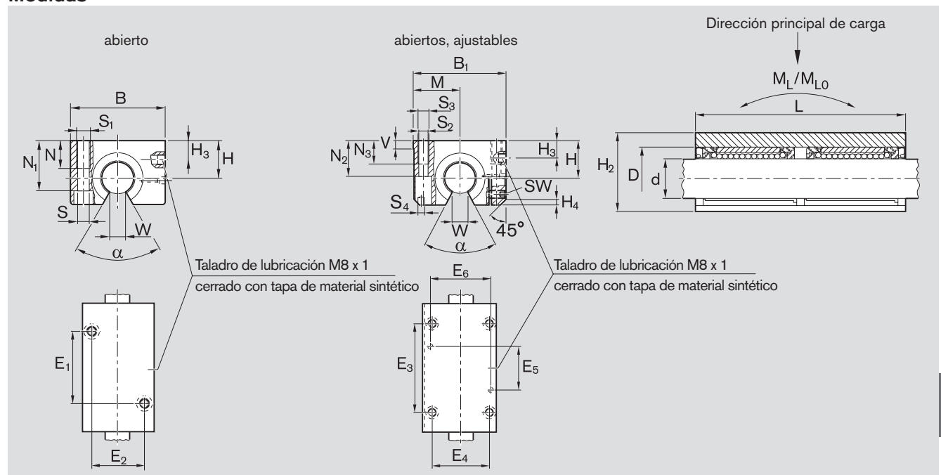
Medidas (mm)
