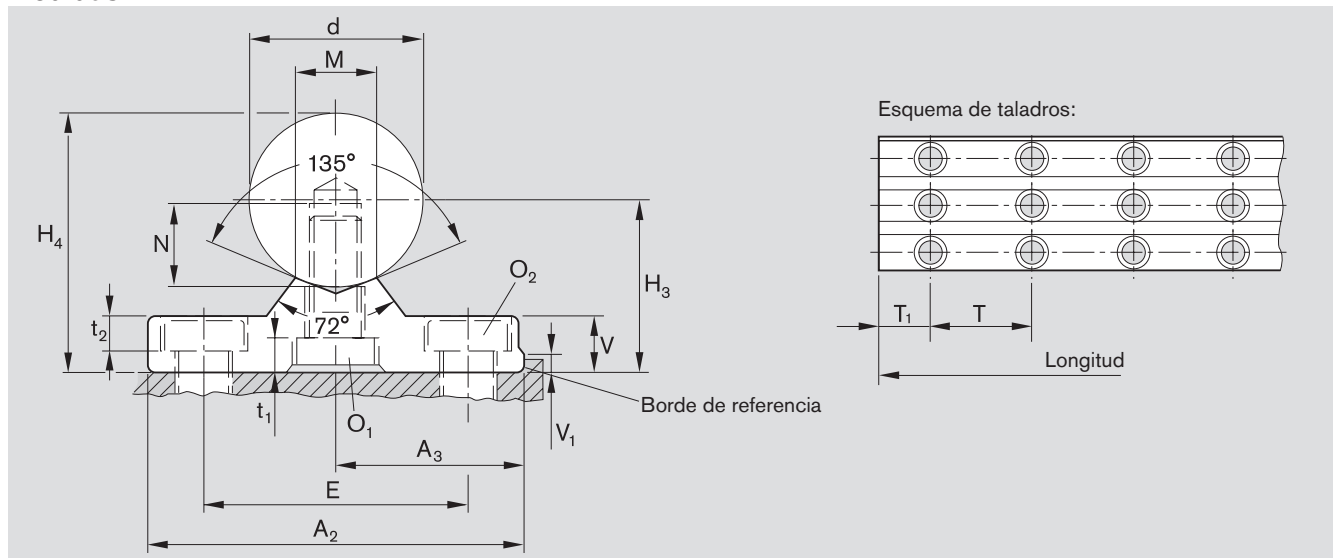
Medidas (mm)
