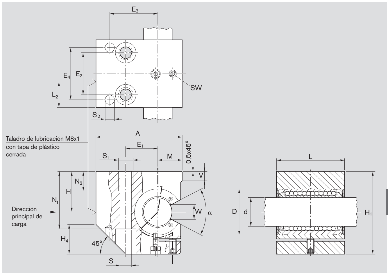
Medidas (mm)
