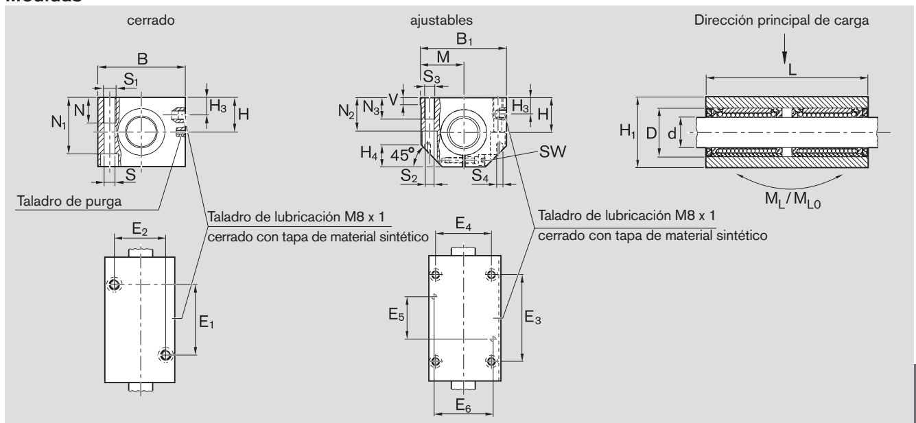
Medidas (mm)
