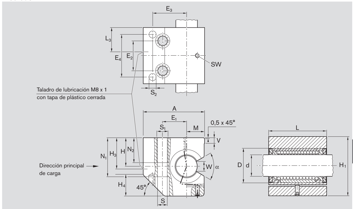
Medidas (mm)
