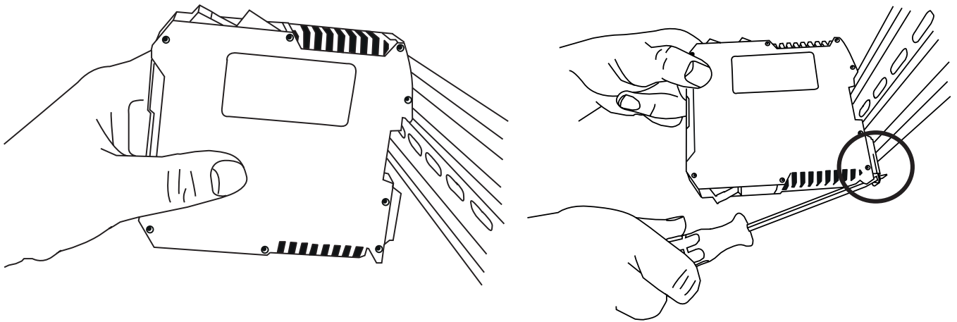
Abb. 1: Montage des VT-MSPA2-2X auf Hutschiene
