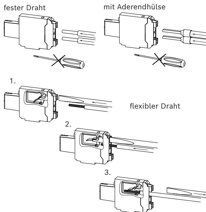
Abb. 3: XG20/XG21: „PUSH-IN“-Kontakt
