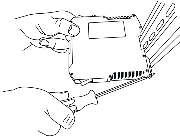
Abb. 6: Demontage des VT-MSPA2-2X von der Hutschiene
