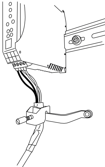
Abb. 2: Schirmung des VT-MSPA2-2X
