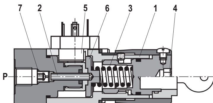
形式 HED 8 OA-2X/...K14KW
