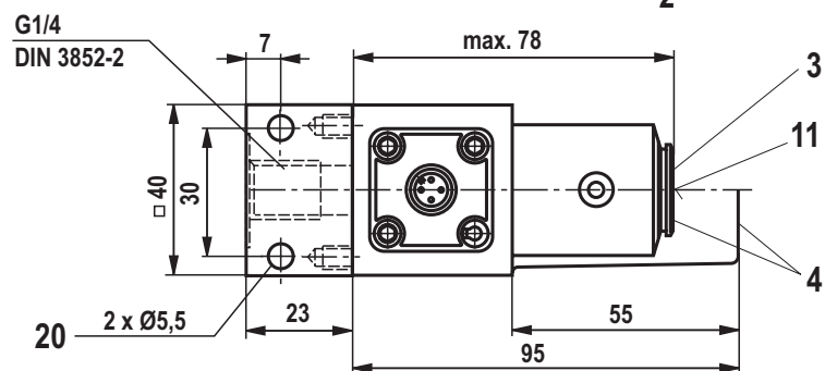
形式 HED 8 OA...
