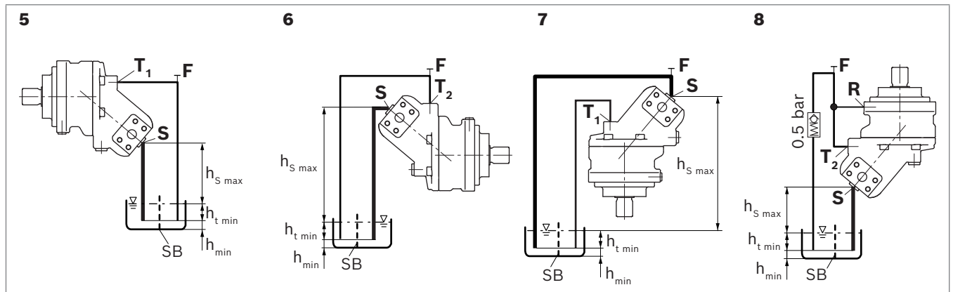
Abb. 8: Übertankeinbau A2FO mit Einbaulage 5–8
