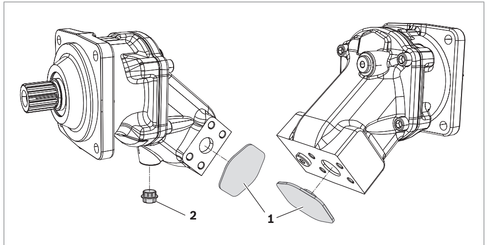
Abb. 1: Axialkolbeneinheit
