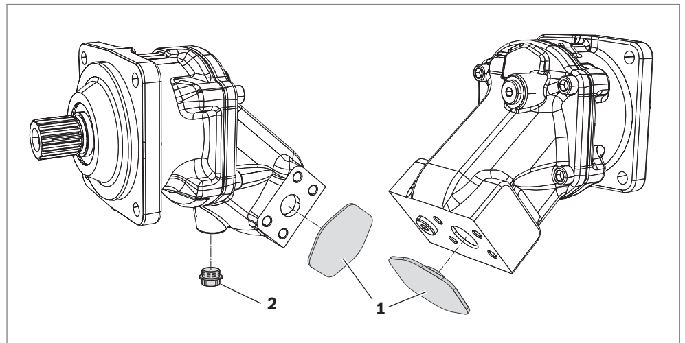
Abb. 10: Transportschutz entfernen
