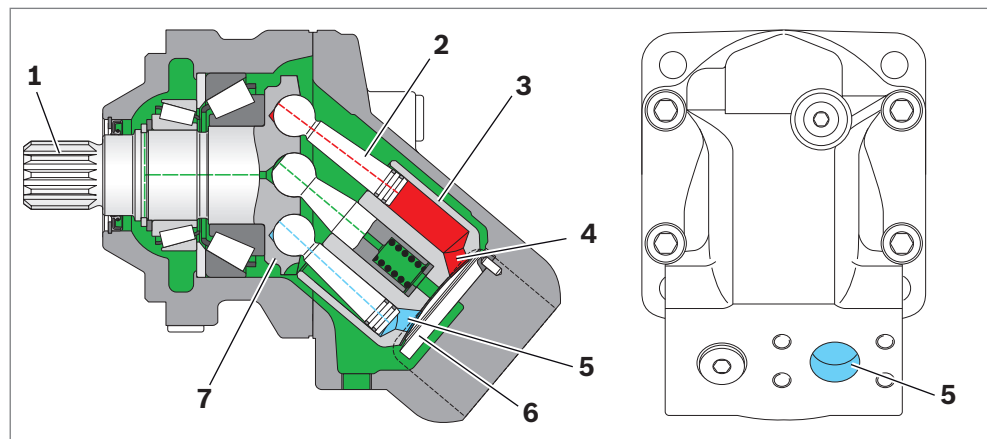
Abb. 2: Aufbau der A2FO Baureihe 70
