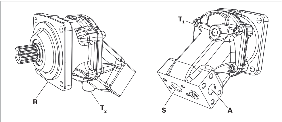
Abb. 12: Anschlussübersicht A2FO, Drehrichtung links
