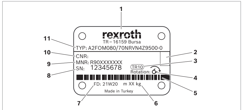
Abb. 3: Typschild A2FO
