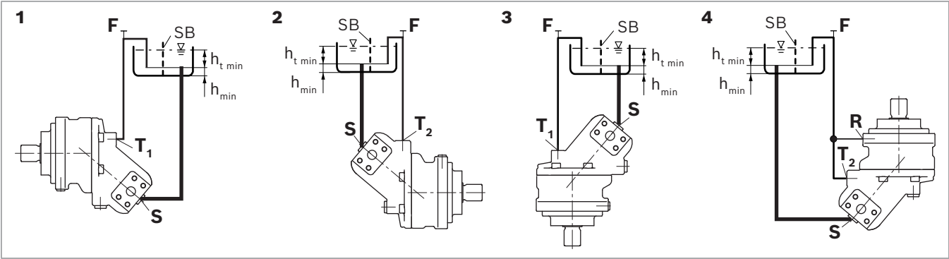
Abb. 7: Untertankeinbau A2FO mit Einbaulage 1–4
