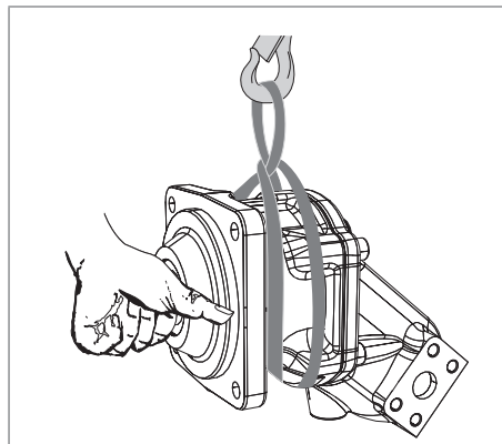
Abb. 5: Transport mit Hebeband
