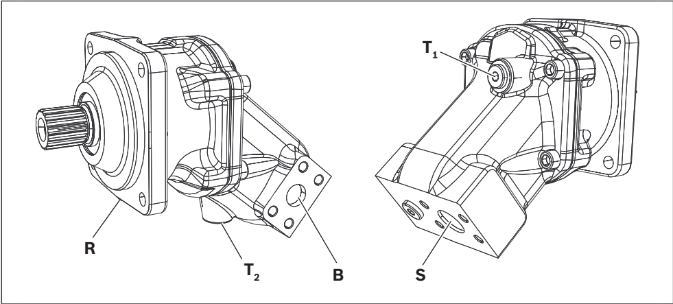
Abb. 11: Anschlussübersicht A2FO, Drehrichtung rechts
