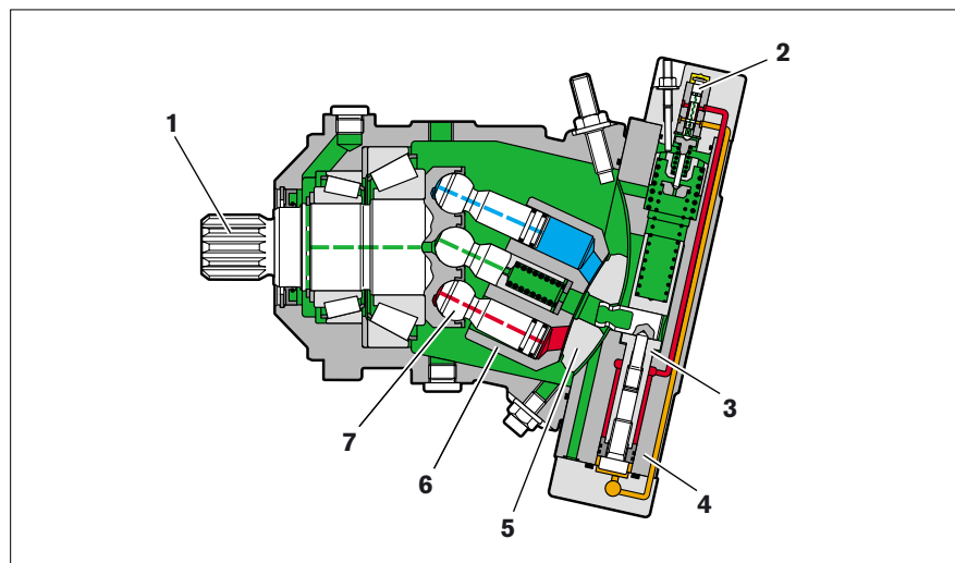
Abb. 2: Aufbau der A6VM
