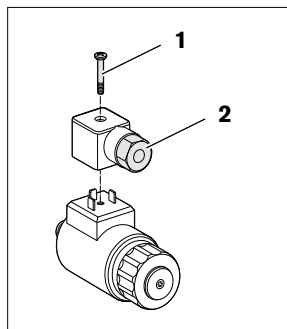
Abb. 19: Anziehdrehmoment Hirschmann-Stecker
