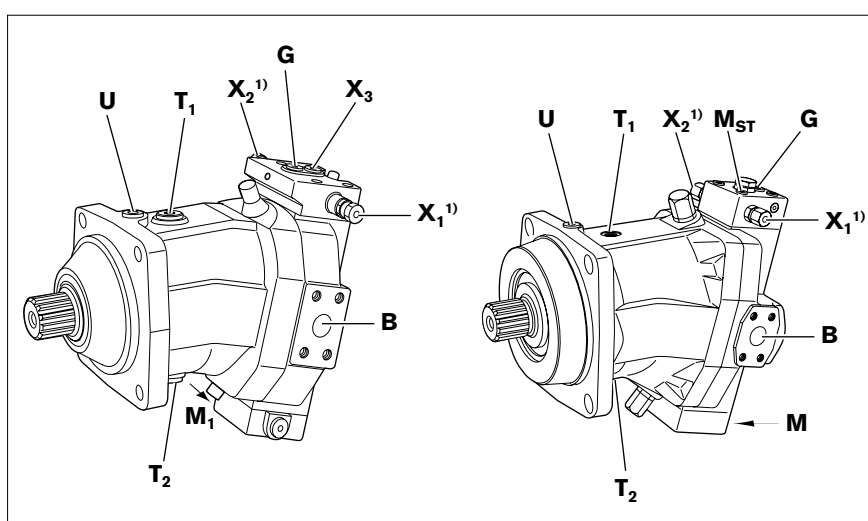
Abb. 18: Anschlussübersicht A6VM 28-200 DA1 (links), A6VM 250-1000 DA (rechts), Arbeitsanschlüsse seitlich
