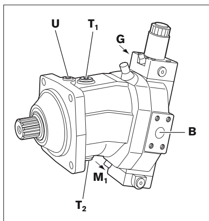
Abb. 16: Anschlussübersicht A6VM 28-200 EP, Arbeitsanschlüsse seitlich
