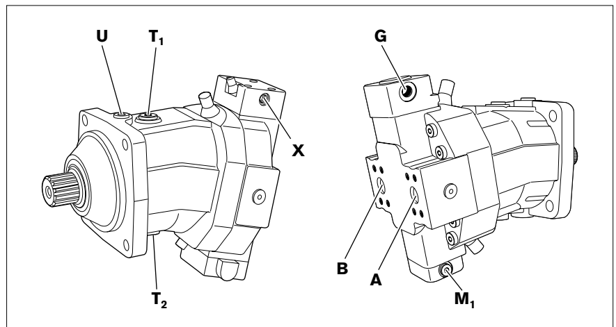
Abb. 12: Anschlussübersicht A6VM 28-200 HD, Arbeitsanschlüsse hinten
