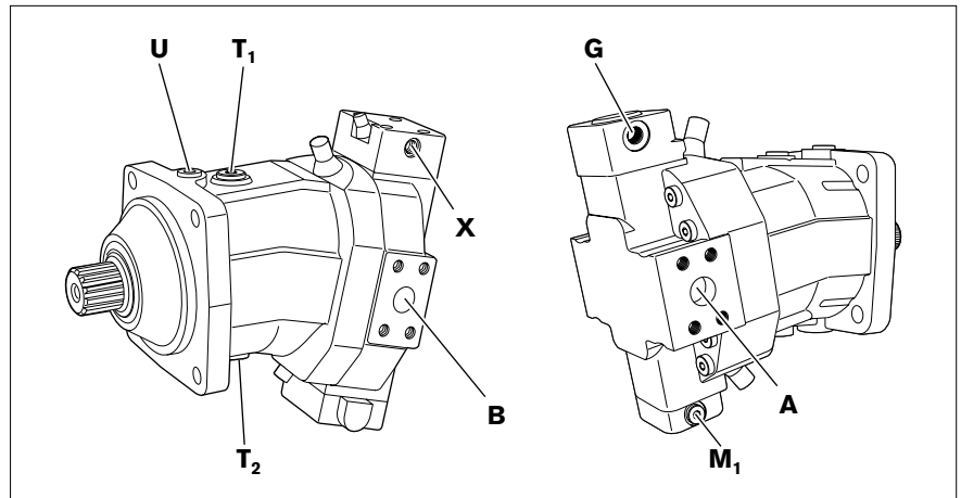
Abb. 11: Anschlussübersicht A6VM 28-200 HD, Arbeitsanschlüsse seitlich
