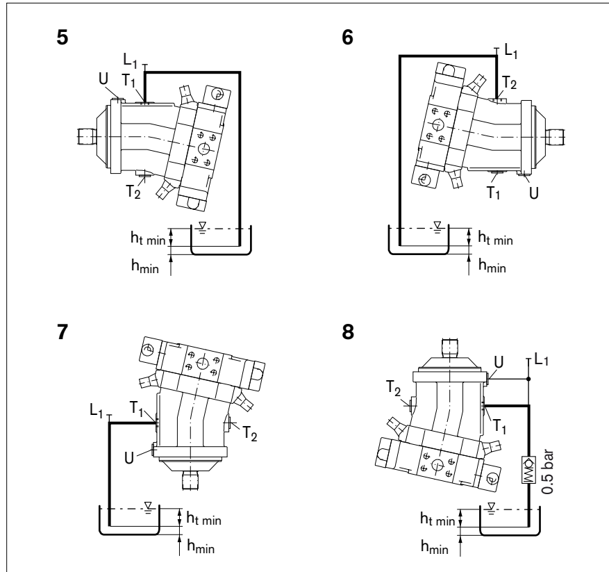
Abb. 7: Übertankeinbau A6VM mit Einbaulage 5–8
