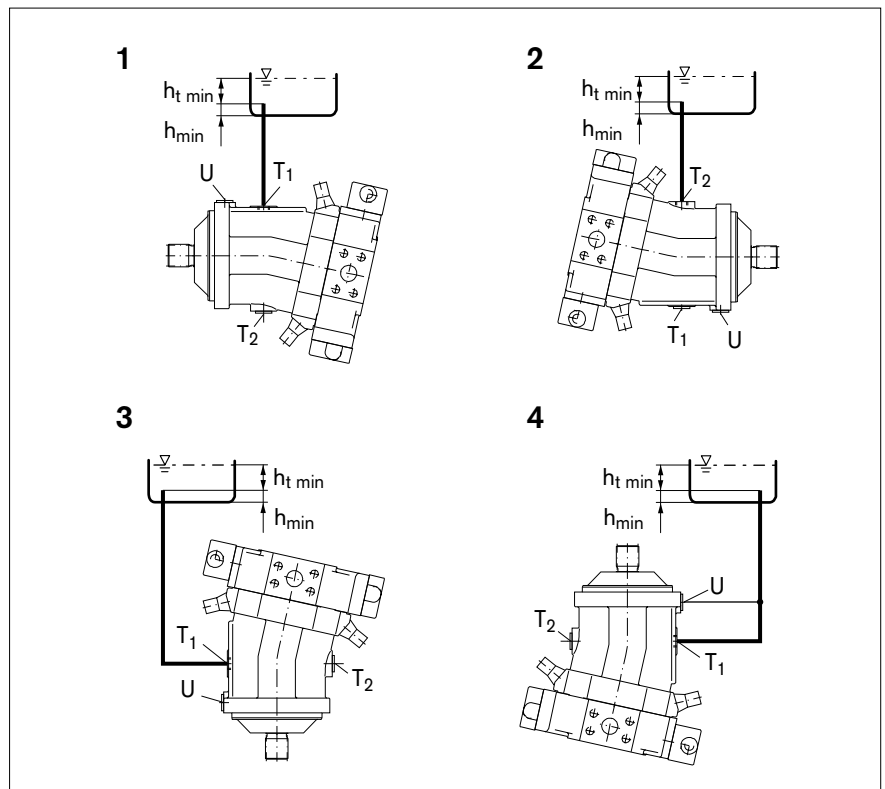
Abb. 6: Untertankeinbau A6VM mit Einbaulage 1–4
