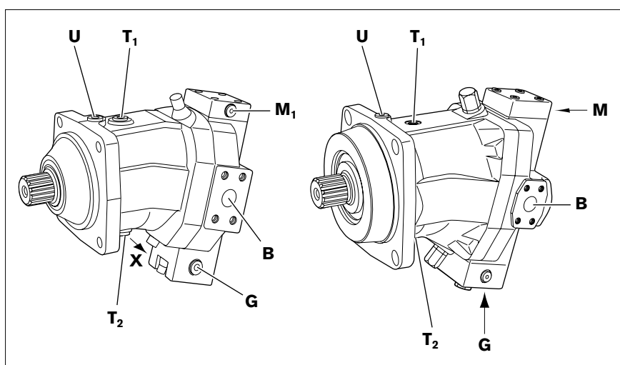
Abb. 17: Anschlussübersicht A6VM 28-200 HA (links), A6VM 250-1000 HA (rechts), Arbeitsanschlüsse seitlich
