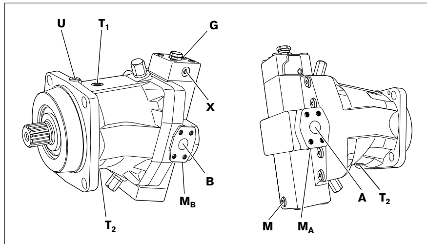
Abb. 13: Anschlussübersicht A6VM 250-1000 HD, Arbeitsanschlüsse seitlich
