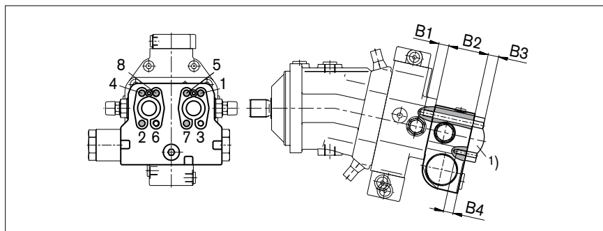
Abb. 10: Befestigung des Bremsventils
