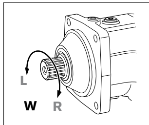
Abb. 8: Drehrichtung
