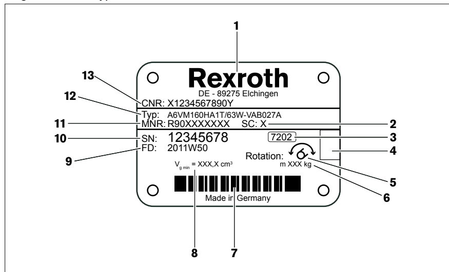
Abb. 3: Typschild A6VM
