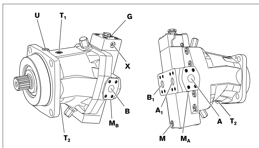
Abb. 15: Anschlussübersicht A6VM 250-1000 HD, Arbeitsanschlüsse seitlich und hinten
