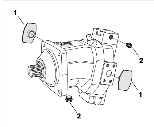
Abb. 9: Transportschutz entfernen
