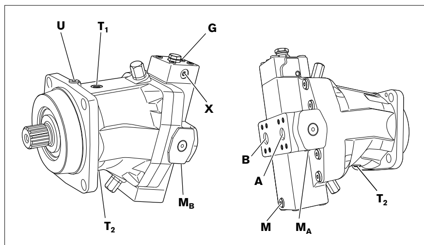
Abb. 14: Anschlussübersicht A6VM 250-1000 HD, Arbeitsanschlüsse hinten
