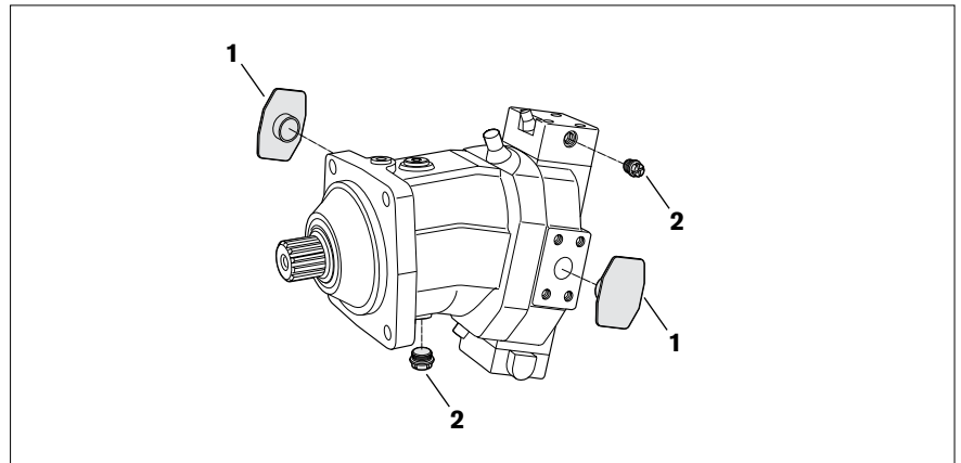
Abb. 1: Axialkolbeneinheit
