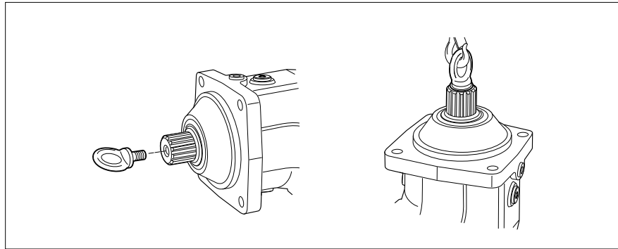
Abb. 4: Befestigung der Ringschraube
