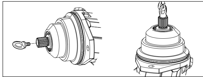
Abb. 4: Befestigung der Ringschraube
