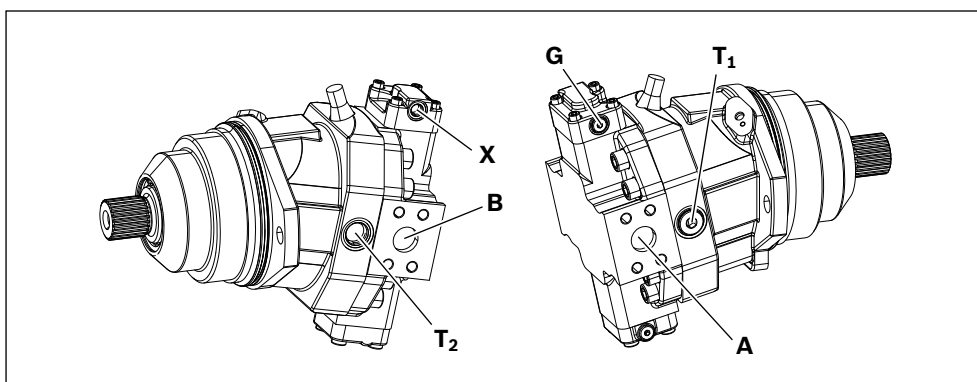
Abb. 13: Anschlussübersicht A6VE mit Verstellung HZ5, Arbeitsanschlüsse seitlich
