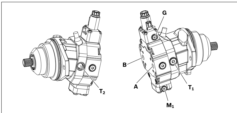
Abb. 11: Anschlussübersicht A6VE mit Verstellung EP5/EP6, Arbeitsanschlüsse hinten
