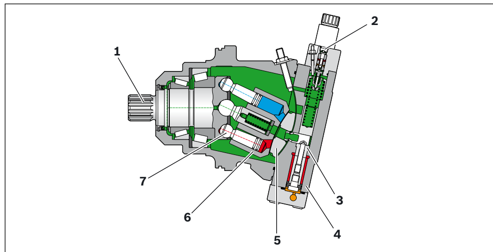
Abb. 2: Aufbau der A6VE
