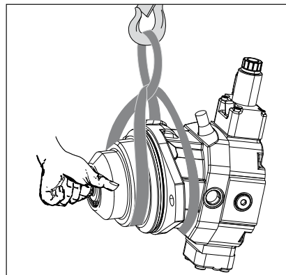
Abb. 5: Transport mit Hebeband
