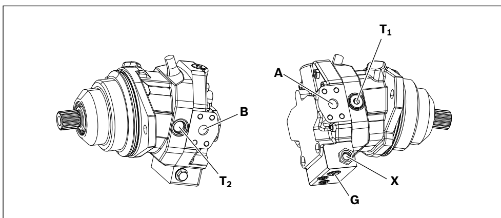
Abb. 12: Anschlussübersicht A6VE mit Verstellung HZ7, Arbeitsanschlüsse seitlich
