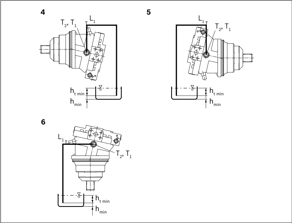
Abb. 7: Übertankeinbau A6VE mit Einbaulage 4–6
