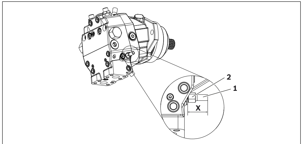
Abb. 15: Integriertes Gegenhalteventil mit Bremslüftventil
