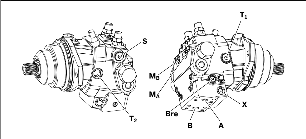
Abb. 14: Anschlussübersicht A6VE mit Verstellung HZ7 und integriertem Gegenhalteventil (BVI), Arbeitsanschlüsse unten
