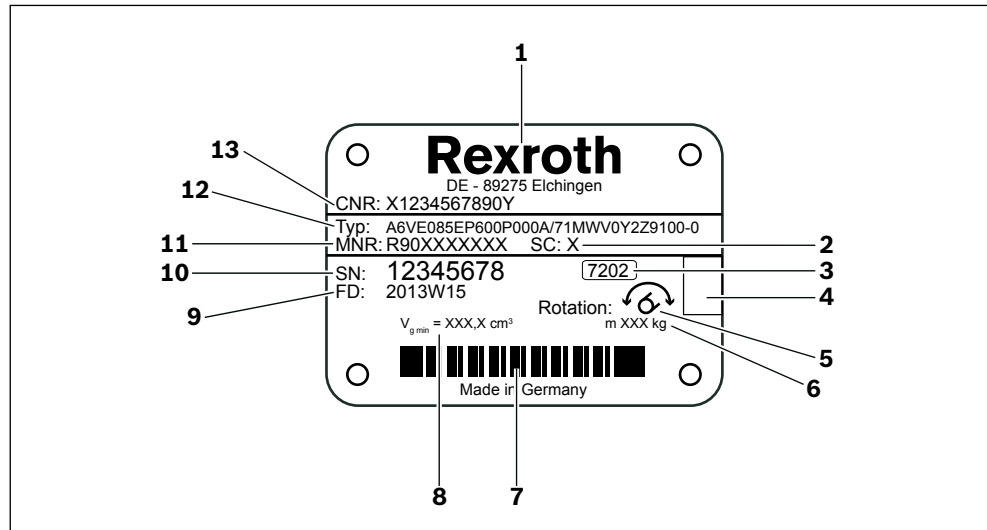
Abb. 3: Typschild A6VE
