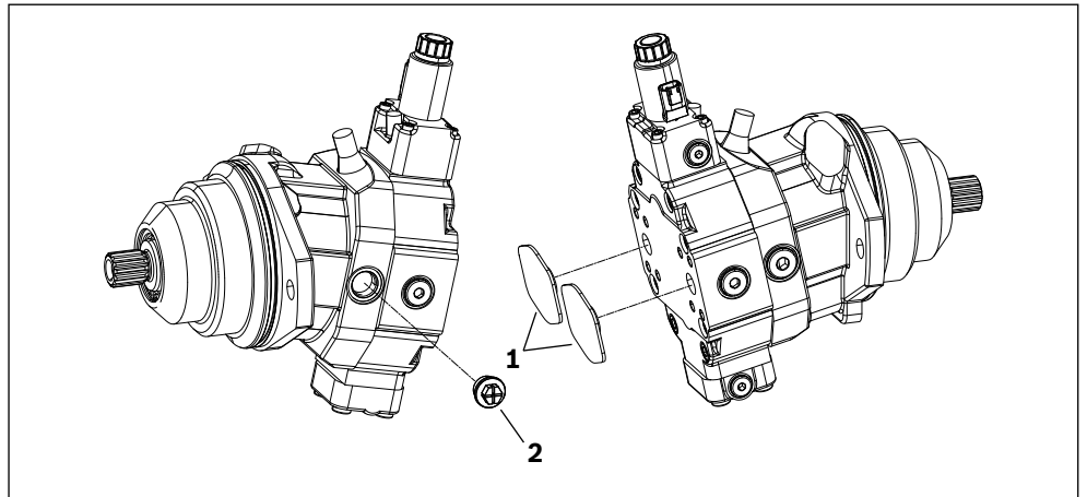
Abb. 1: Axialkolbeneinheit
