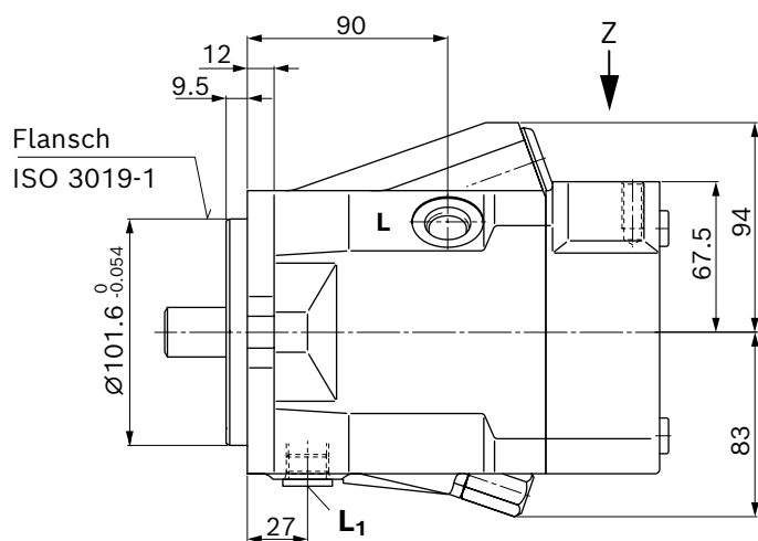
Anschlussplatte 10 (60)
