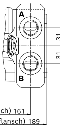
Teilansicht Z
