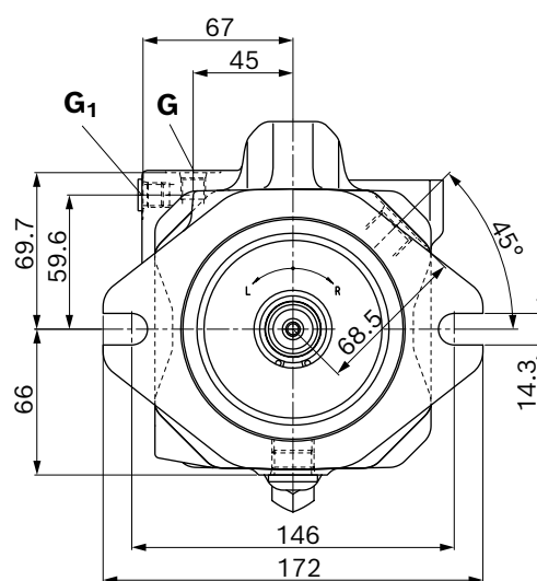
Anschlussplatte 16 (66)
