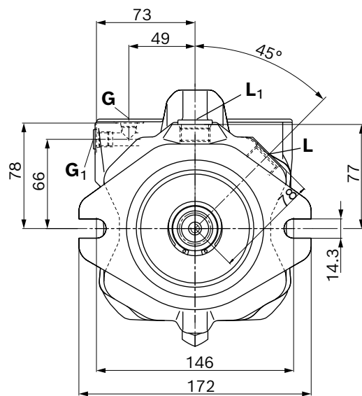
Ansicht Z Anschlussplatte 11 (61)
