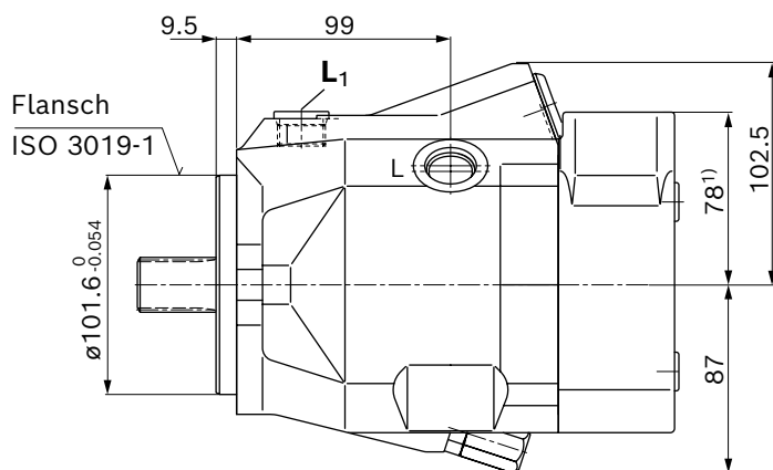
Anschlussplatte 10 (60)
