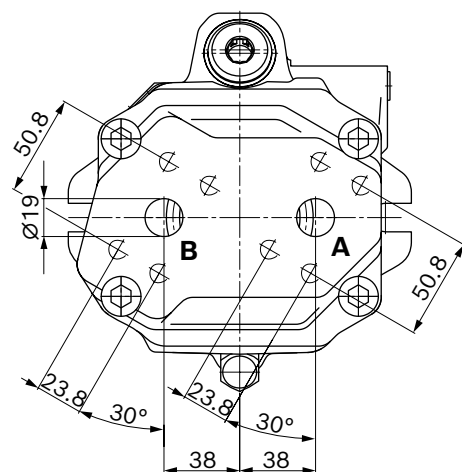
Ansicht Z Anschlussplatte 11 (61)
