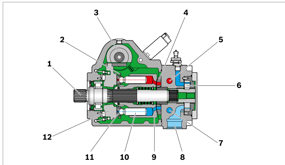
Abb. 2: Aufbau der A4VG Baureihe 35
