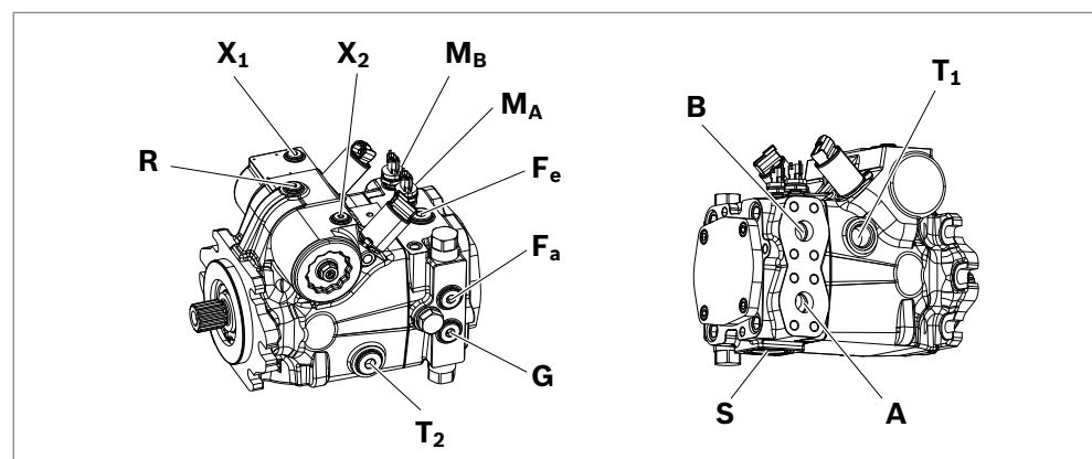
Abb. 13: Anschlussübersicht A4VG
