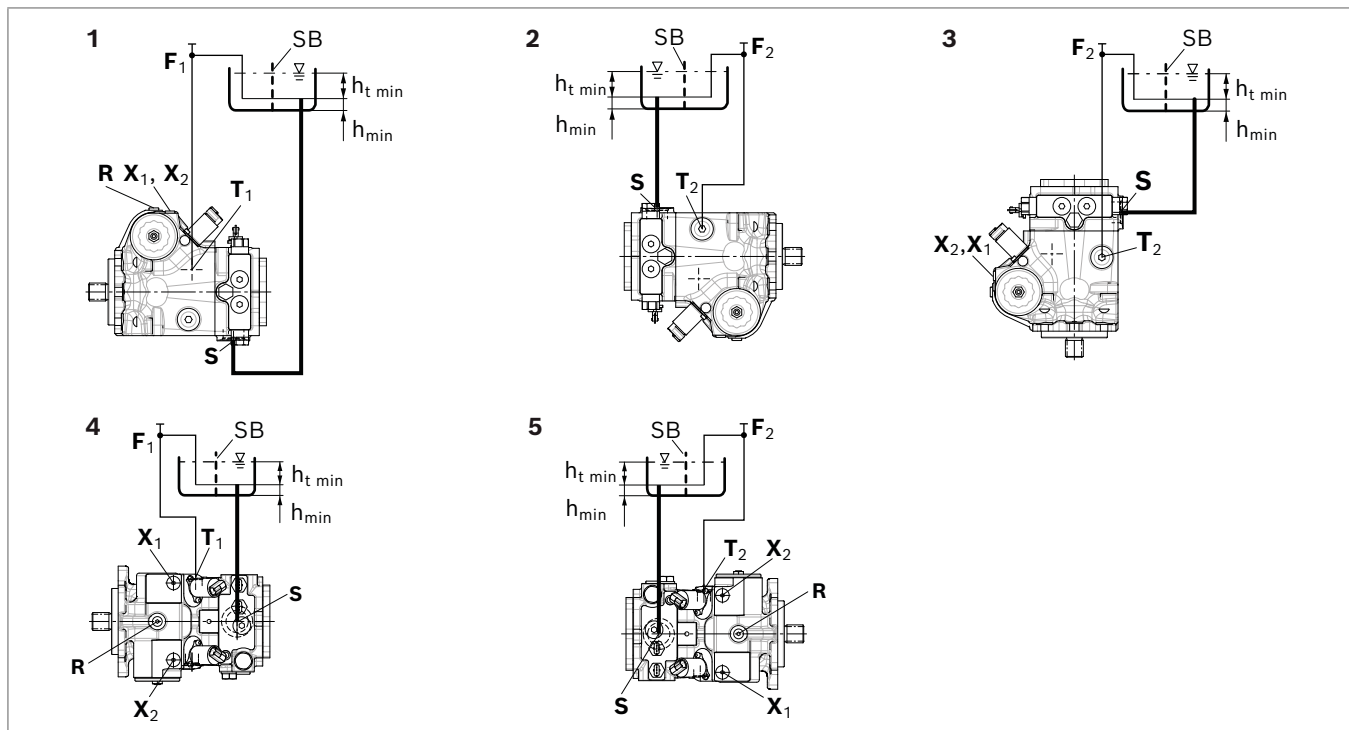
Abb. 9: Untertankeinbau A4VG mit Einbaulage 1–5
