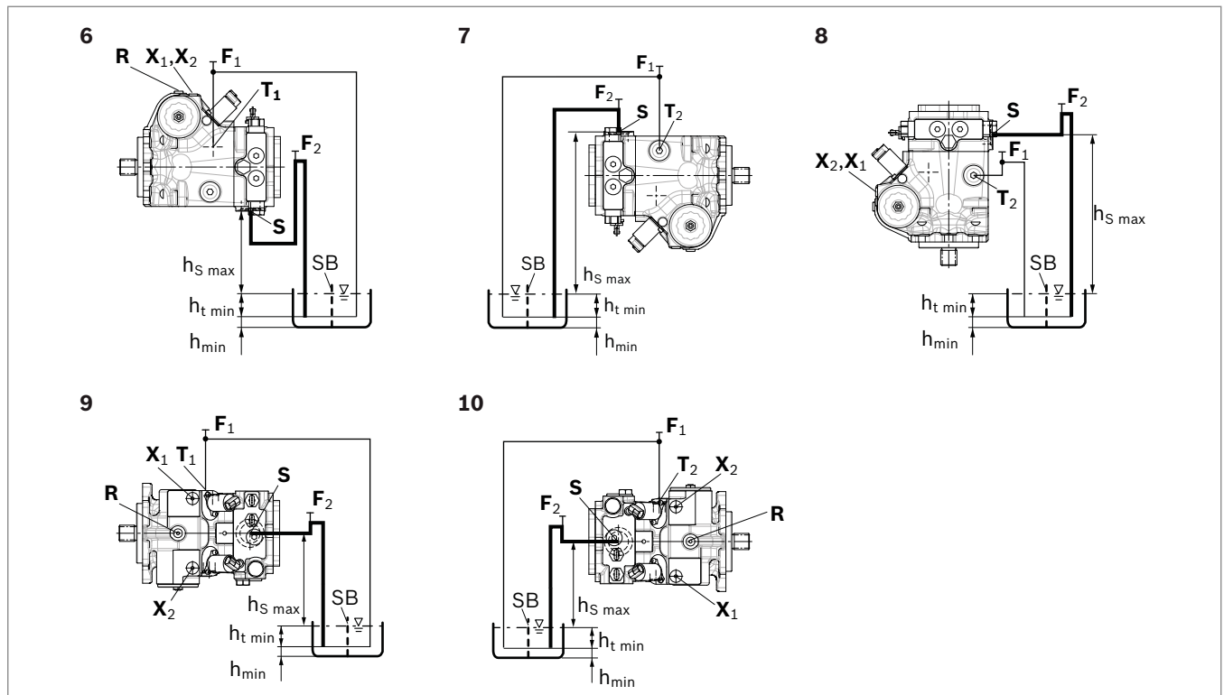
Abb. 10: Übertankeinbau A4VG mit Einbaulage 6–10
