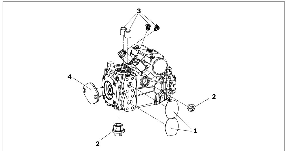
Abb. 1: Axialkolbeneinheit
