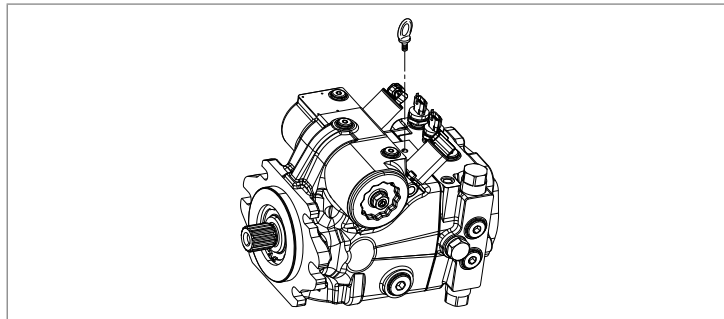
Abb. 6: Befestigung der Ringschraube im Gehäuse
