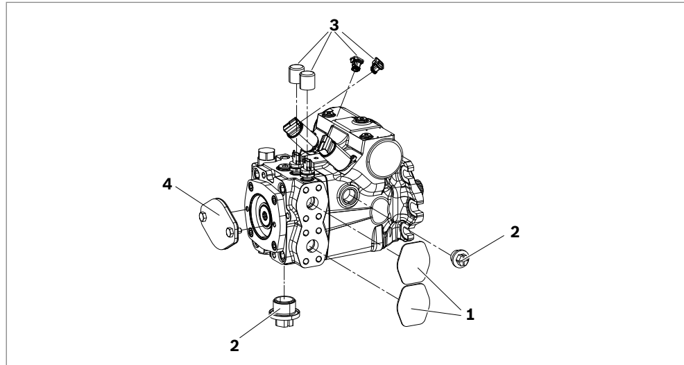
Abb. 12: Transportschutz entfernen
