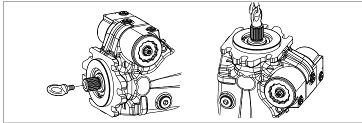
Abb. 5: Befestigung der Ringschraube
