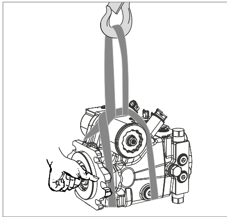
Abb. 7: Transport mit Hebeband
