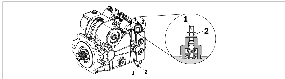
Abb. 3: Bypass-Funktion aktivieren
