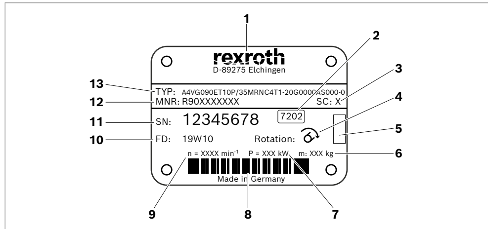
Abb. 4: Typschild A4VG
