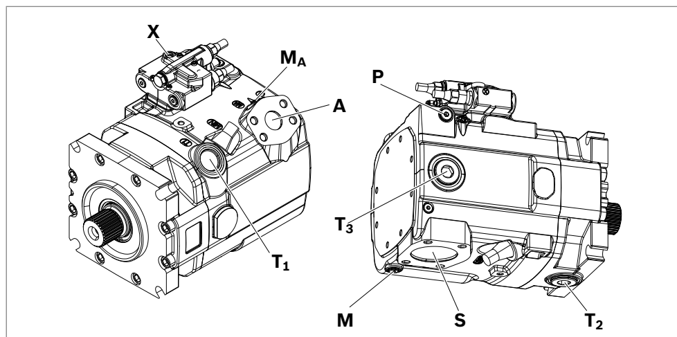
Abb. 15: Anschlussübersicht A15VO mit LRDRS.-Regler, Drehrichtung rechts
