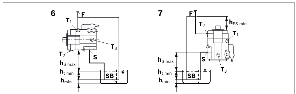
Abb. 11: Übertankeinbau A15VO/A15VLO mit Einbaulage 6–7
