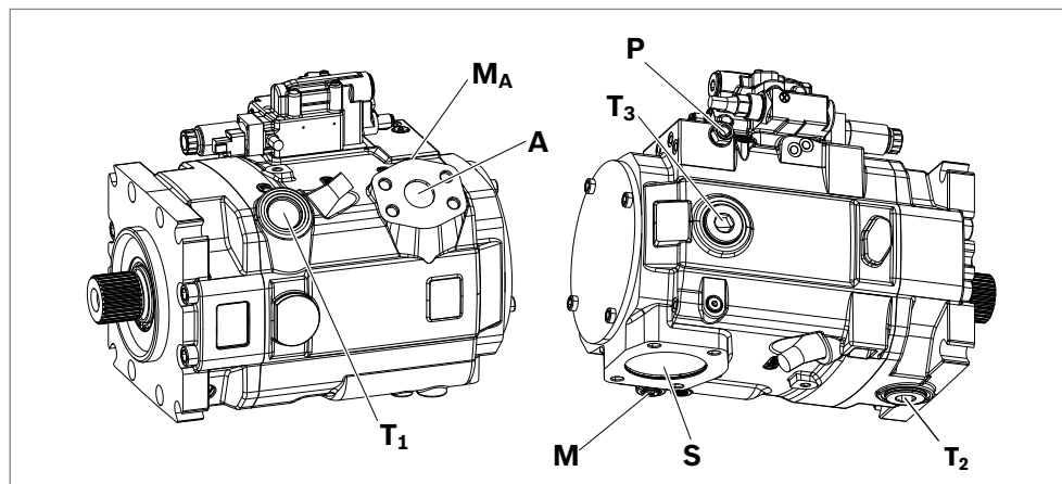
Abb. 14: Anschlussübersicht A15VLO mit E2DR-Regler, Drehrichtung rechts
