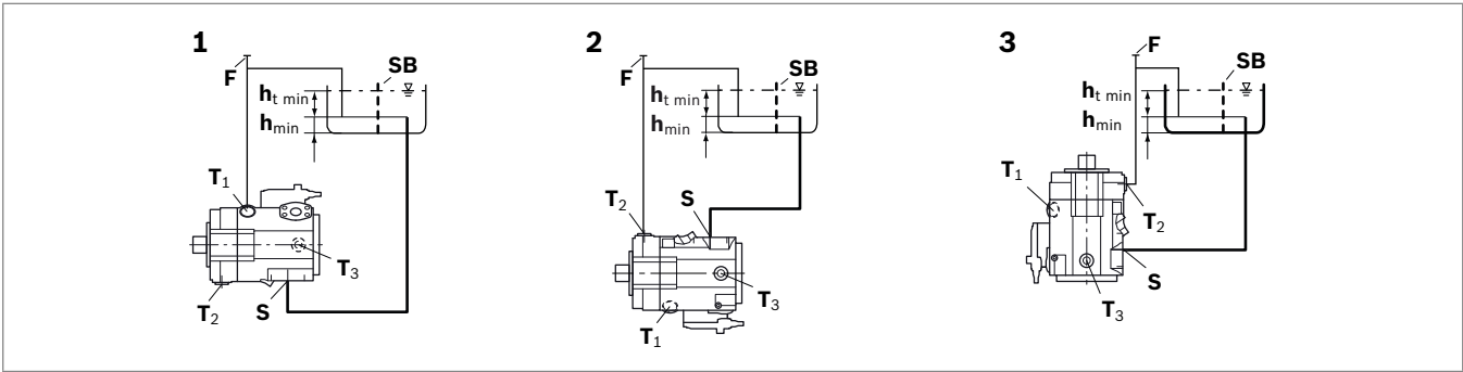
Abb. 9: Untertankeinbau A15VO/A15VLO mit Einbaulage 1–3
