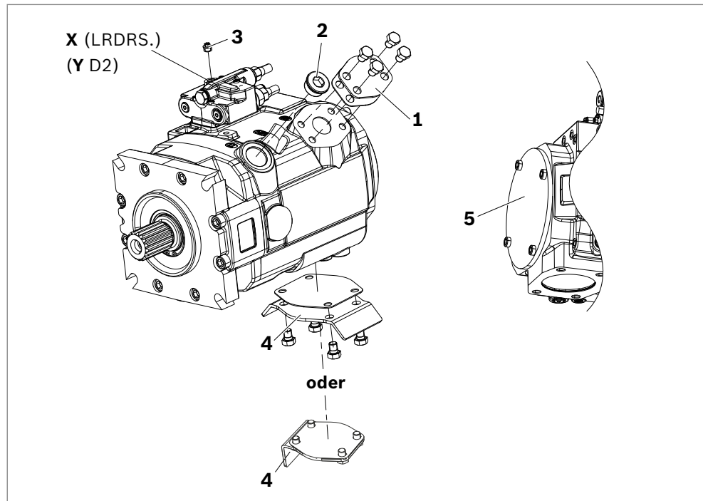
Abb. 13: Transportschutz entfernen
