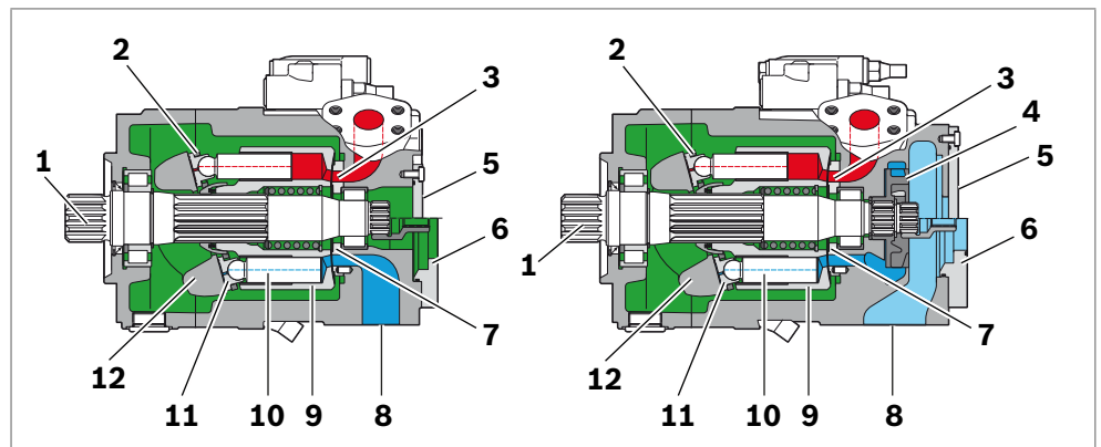
Abb. 2: Linke Darstellung: Aufbau der A15VO; rechte Darstellung: Aufbau der A15VLO
