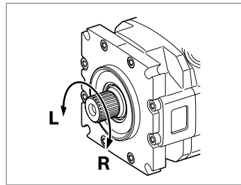
Abb. 12: Drehrichtung
