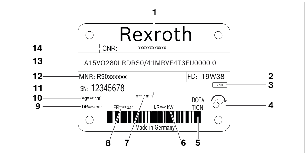
Abb. 4: Typschild A15V(L)O
