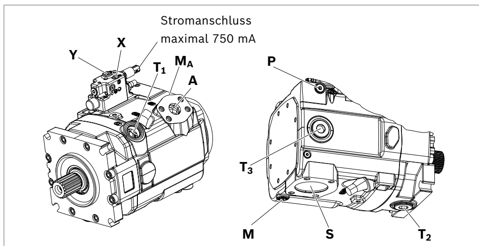
Abb. 17: Anschlussübersicht D2 Regler, Drehrichtung rechts
