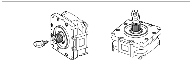
Abb. 5: Befestigung der Ringschraube in der Triebwelle
