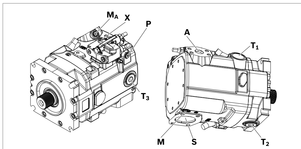
Abb. 16: Anschlussübersicht A15VO mit LRDRS.-Regler, Drehrichtung links
