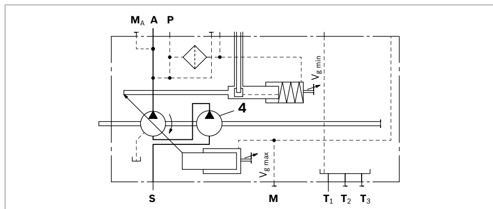
Abb. 3: Schaltplan A15VLO mit Ladepumpe
