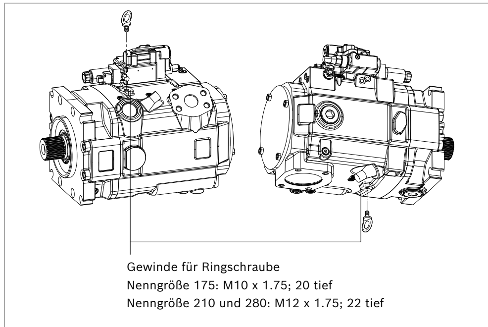
Abb. 6: Befestigung der Ringschraube im Gehäuse oben oder unten
