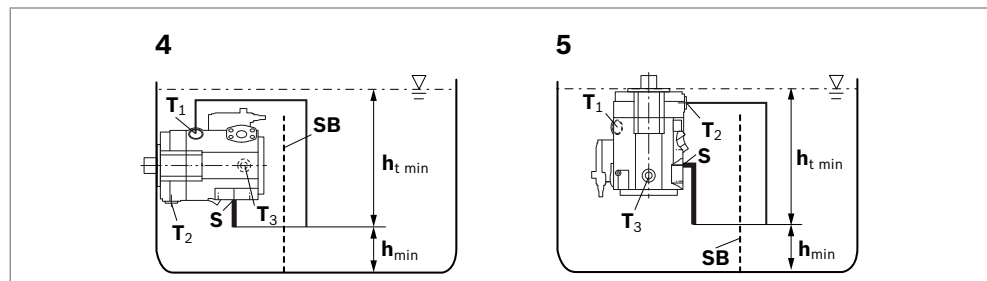
Abb. 10: Tankeinbau A15VO/A15VLO mit Einbaulage 4–5
