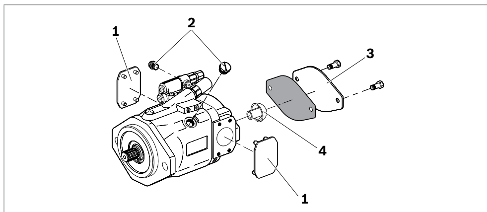
Abb. 12: Transportschutz entfernen
