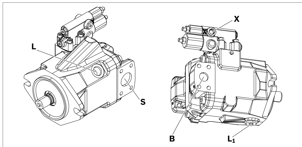
Abb. 14: Anschlussübersicht A10VO/52, SAE Flanschanschlüsse seitlich (Anschlussplatte 12)
