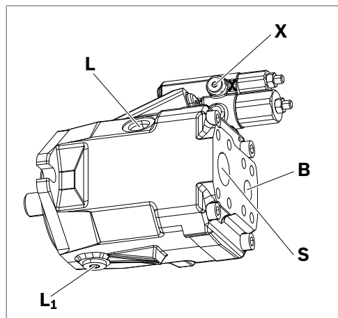
Abb. 13: Anschlussübersicht A10VO/52 bzw. A10VNO/52, SAE Flanschanschlüsse hinten (Anschlussplatte 11)
