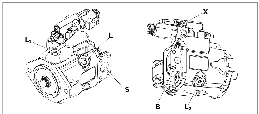
Abb. 17: Anschlussübersicht A10VO/53, SAE Flanschanlüsse seitlich (Anschlussplatte 12)
