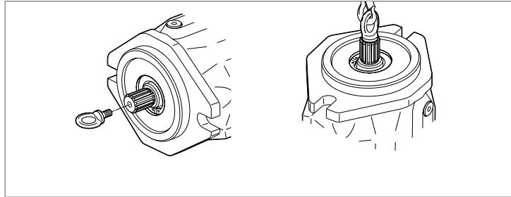
Abb. 4: Befestigung der Ringschraube
