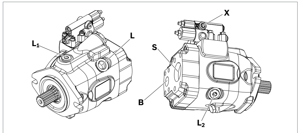
Abb. 16: Anschlussübersicht A10VO/53 bzw. A10VNO/53, SAE Flanschanlüsse hinten (Anschlussplatte 11)
