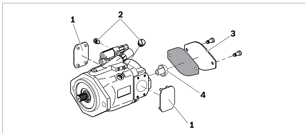
Abb. 1: Axialkolbeneinheit A10VO
