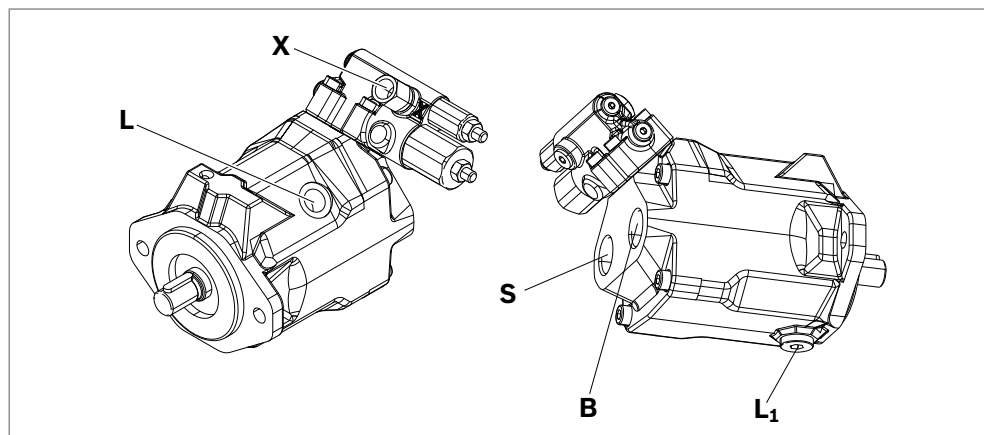
Abb. 15: Anschlussübersicht A10VSO/52 Nenngroße 10 bzw. A10VSNO/52 Nenngroße 15, metrische Gewindeanschlüsse hinten (Anschlussplatte 14)
