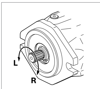
Abb. 10: Drehrichtung
