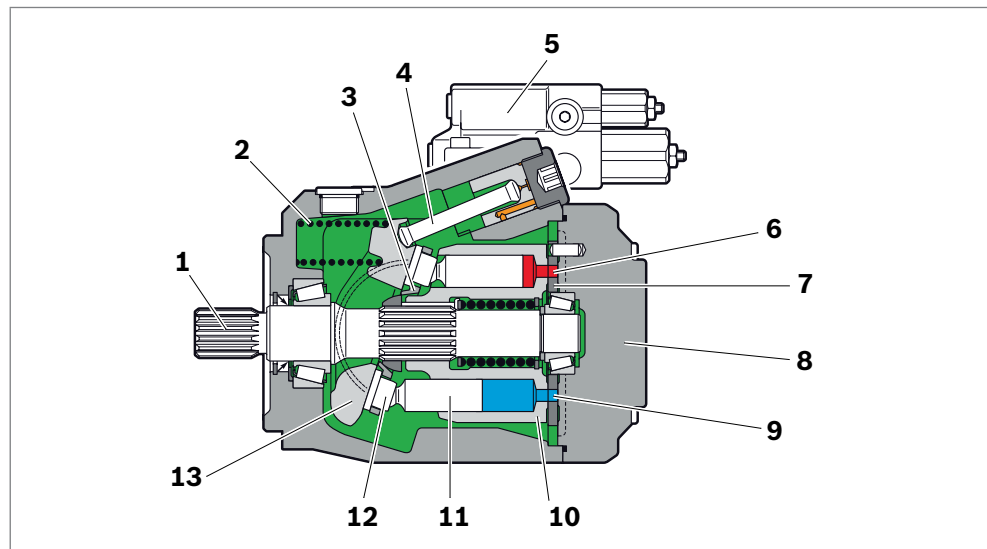
Abb. 2: Aufbau der A10VO
