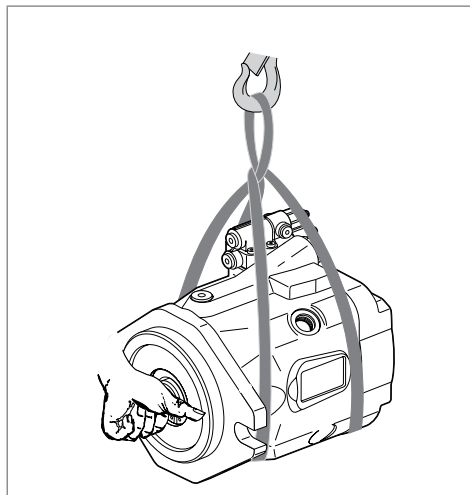
Abb. 5: Transport mit Hebeband
