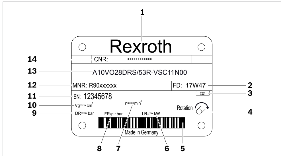
Abb. 3: Typschild A10VO
