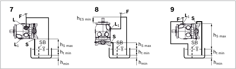
Abb. 9: Übertankeinbau A10VO mit Einbaulage 7–9
