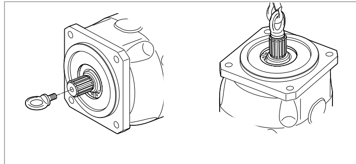
Abb. 4: Befestigung der Ringschraube
