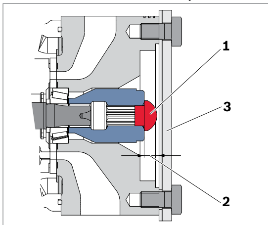
Abb. 11: Distanzhalter entfernen
