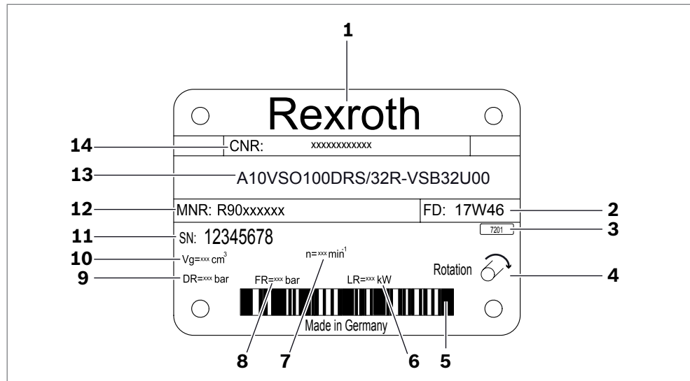
Abb. 3: Typschild A10VSO
