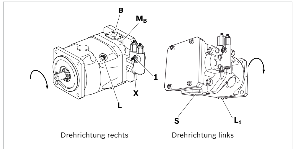
Abb. 13: Anschlussübersicht A10VO, A10VSO und A10VSNO Baureihe 32, SAE-Flanschanschlüsse oben, unten gegenüberliegend
