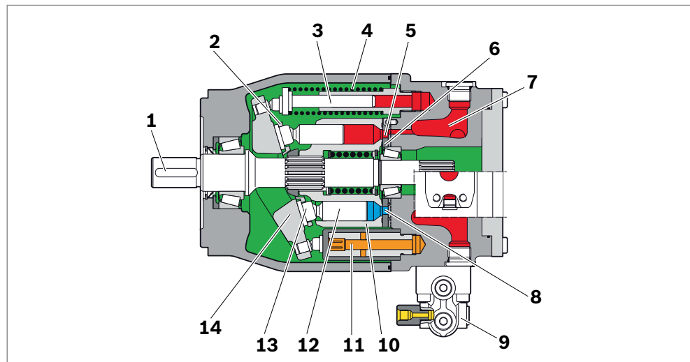
Abb. 2: Aufbau der A10VSO
