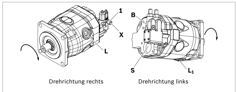
Abb. 14: Anschlussübersicht A10VO Baureihe 32, SAE-Flanschanschlüsse hinten
