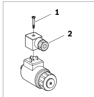
Abb. 15: Hirschmann-Stecker
