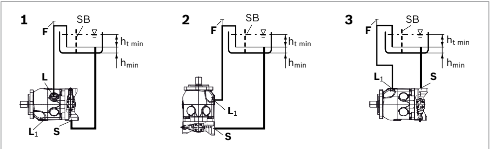
Abb. 7: Untertankeinbau A10VO, A10VSO und A10VSNO mit Einbaulage 1-3
