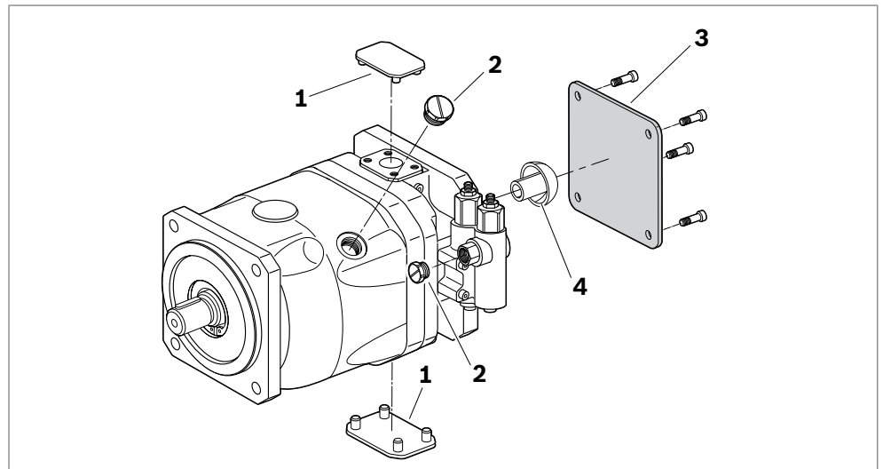
Abb. 1: Axialkolbeneinheit
