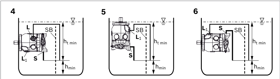
Abb. 8: Tankeinbau
