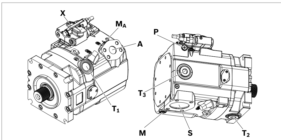
Abb. 15: Anschlussübersicht A15VSO mit LRDRS0-Verstellung, Drehrichtung rechts
