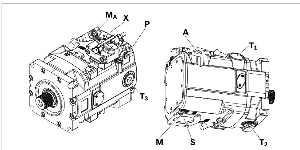
Abb. 16: Anschlussübersicht A15VSO mit LRDRS0-Verstellung, Drehrichtung links
