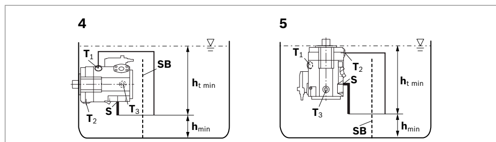
Abb. 10: Tankeinbau A15VSO/A15VLO mit Einbaulage 4–5
