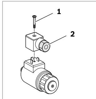
Abb. 17: Hirschmann-Stecker
