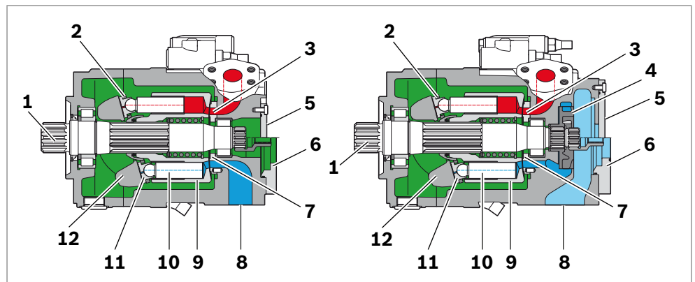
Abb. 2: Linke Darstellung: Aufbau der A15VSO; rechte Darstellung: Aufbau der A15VLO
