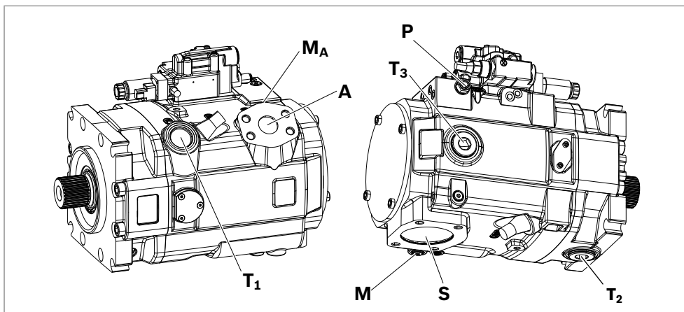
Abb. 14: Anschlussübersicht A15VLO mit E2DR-Verstellung, Drehrichtung rechts
