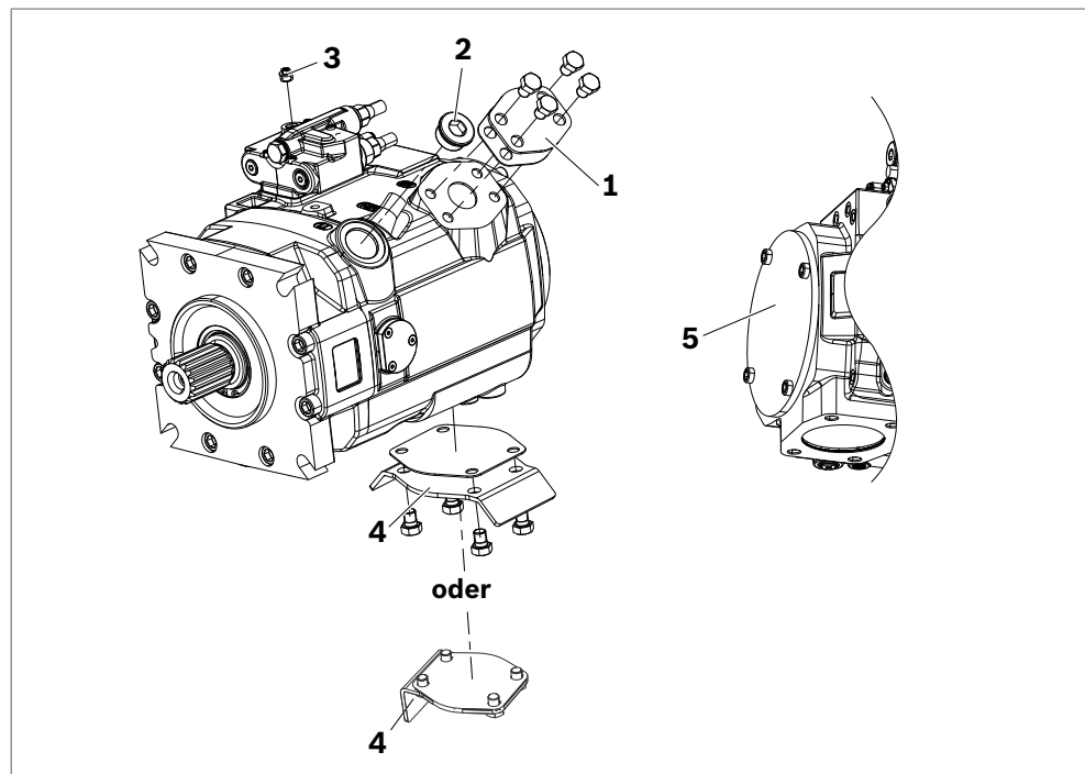
Abb. 1: Axialkolbeneinheit
