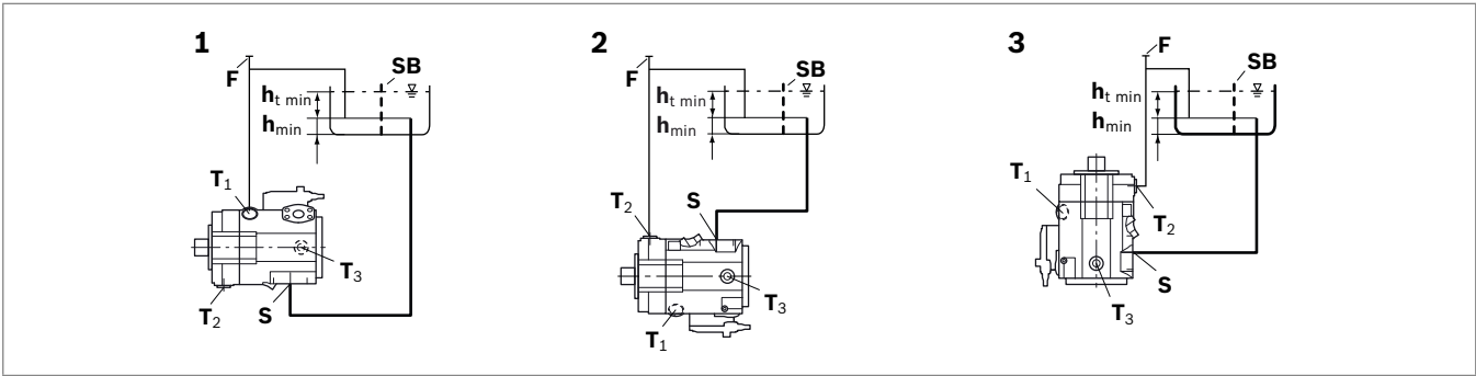
Abb. 9: Untertankeinbau A15VSO/A15VLO mit Einbaulage 1–3
