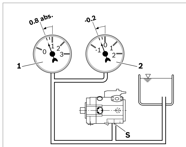
Abb. 8: Saugdruck
