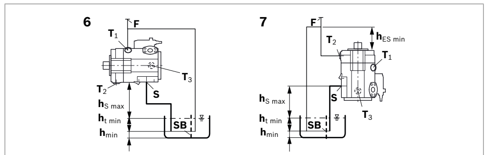
Abb. 11: Übertankeinbau A15VSO/A15VLO mit Einbaulage 6–7
