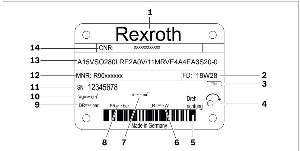
Abb. 4: Typschild A15VSO
