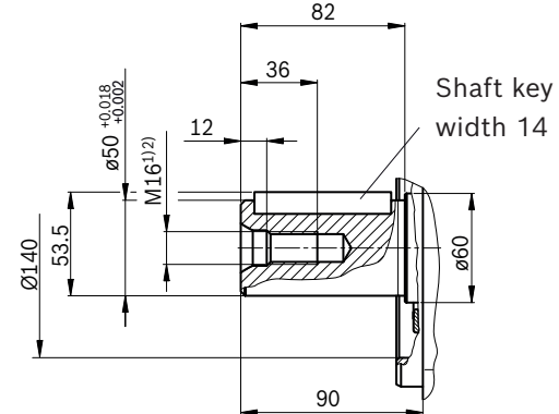
B2 – Ø50 A 14x9x80
