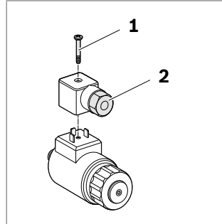
Fig. 15: Connettore Hirschmann
