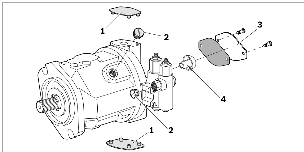
Fig. 12: Rimozione della protezione di trasporto
