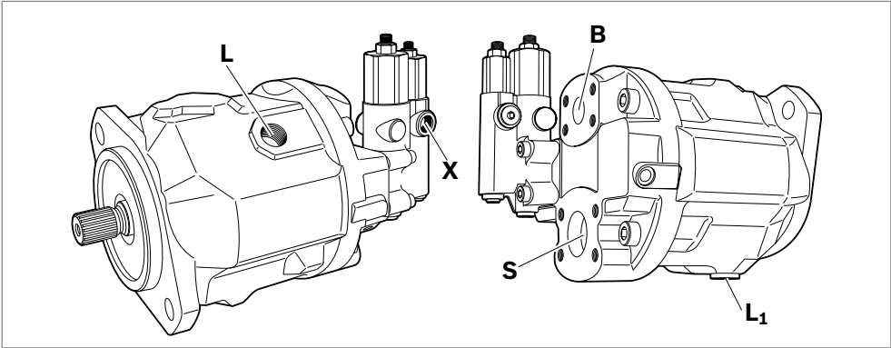
Fig. 13: Panoramica degli attacchi A10VO Serie 31, attacchi flangiati SAE posteriori
