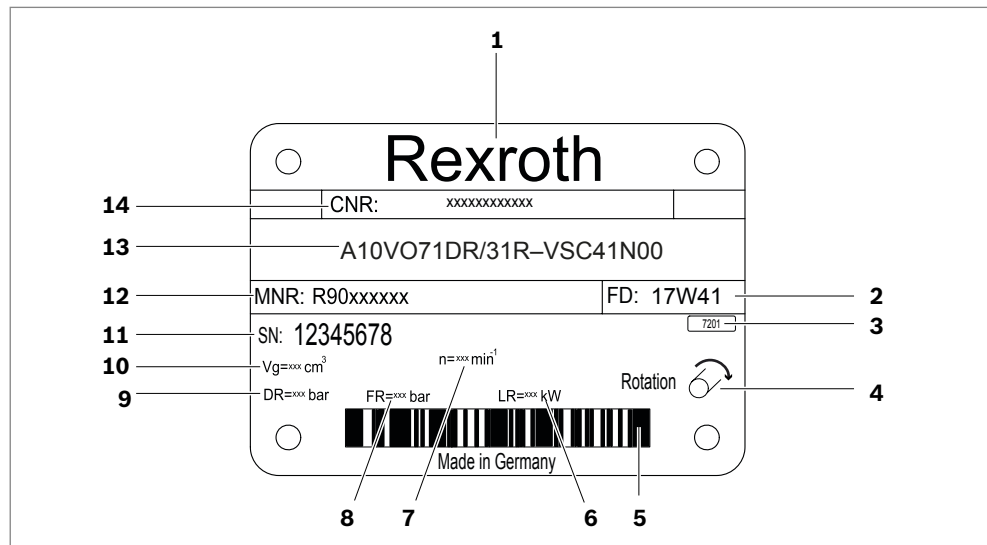
Fig. 3: Targhetta di identificazione A10VO
