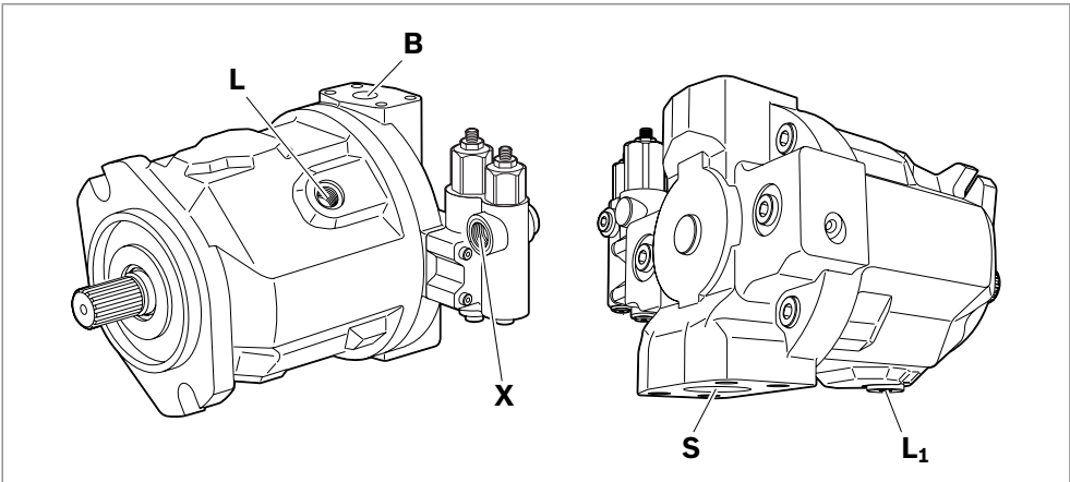
Fig. 14: Panoramica degli attacchi A10VO/A10VSO Serie 31, attacchi flangiati SAE superiori, inferiori contrapposti
