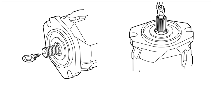
Fig. 4: Fissaggio del golfare ad anello
