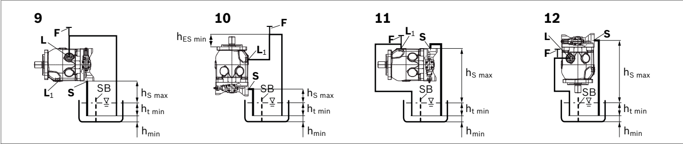
Fig. 9: Montaggio al di sopra del serbatoio A10VO/A10VSO con posizione di montaggio 9-12
