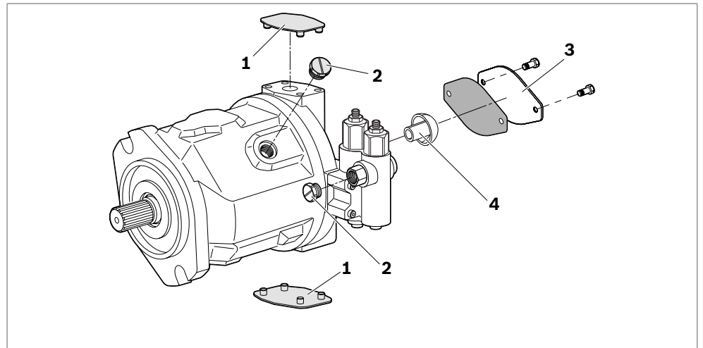
Fig. 1: Unità a pistoni assiali A10VSO
