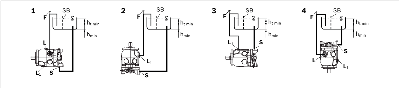
Fig. 7: Montaggio al di sotto del serbatoio A10VO/A10VSO con posizione di montaggio 1–4
