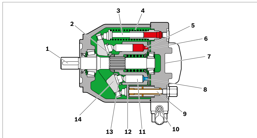
Fig. 2: Struttura dell'A10VO/A10VSO
