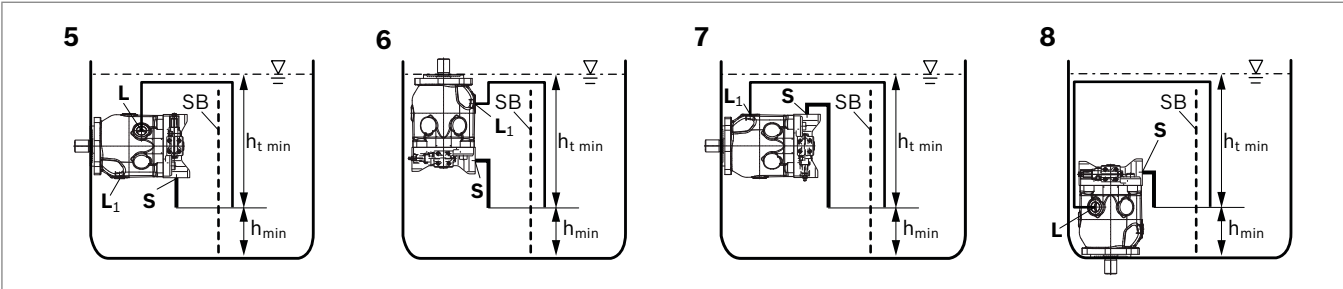
Fig. 8: Montaggio all'interno del serbatoio A10VO/A10VSO con posizione di montaggio 5-8
