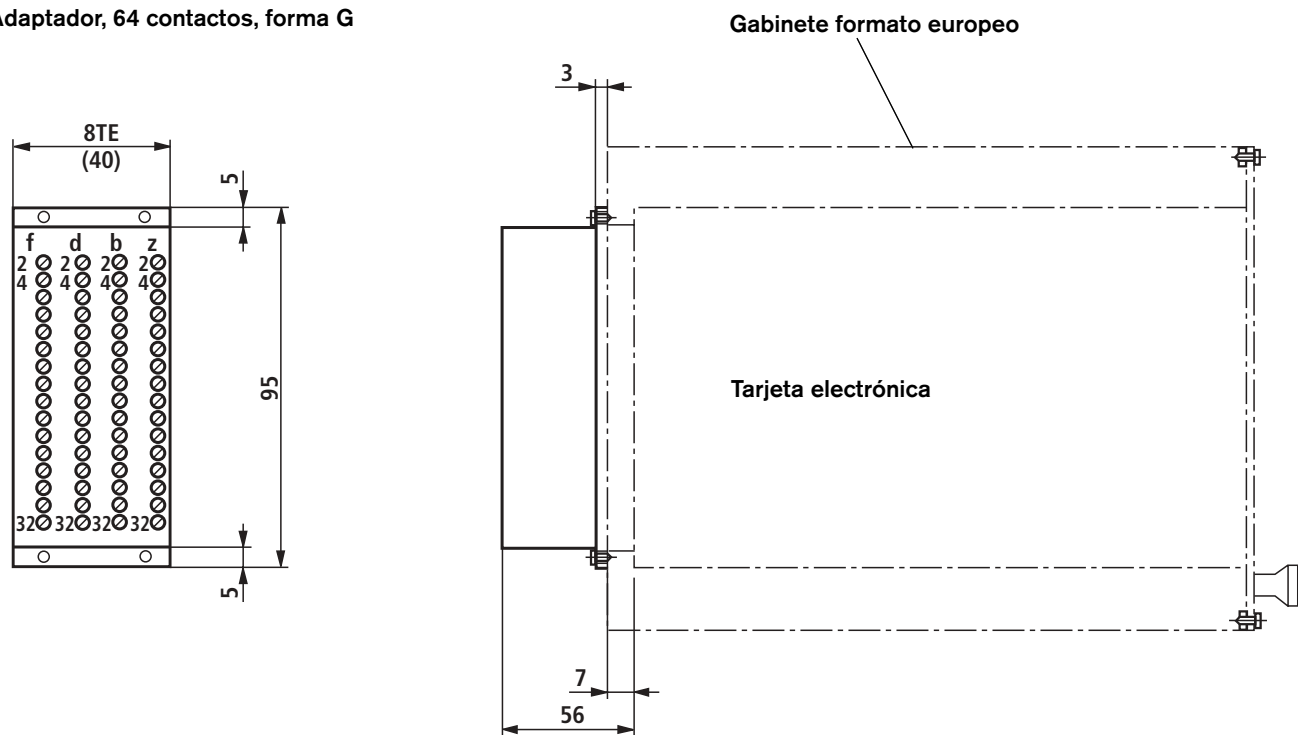
Adaptador, 64 contactos, forma G
