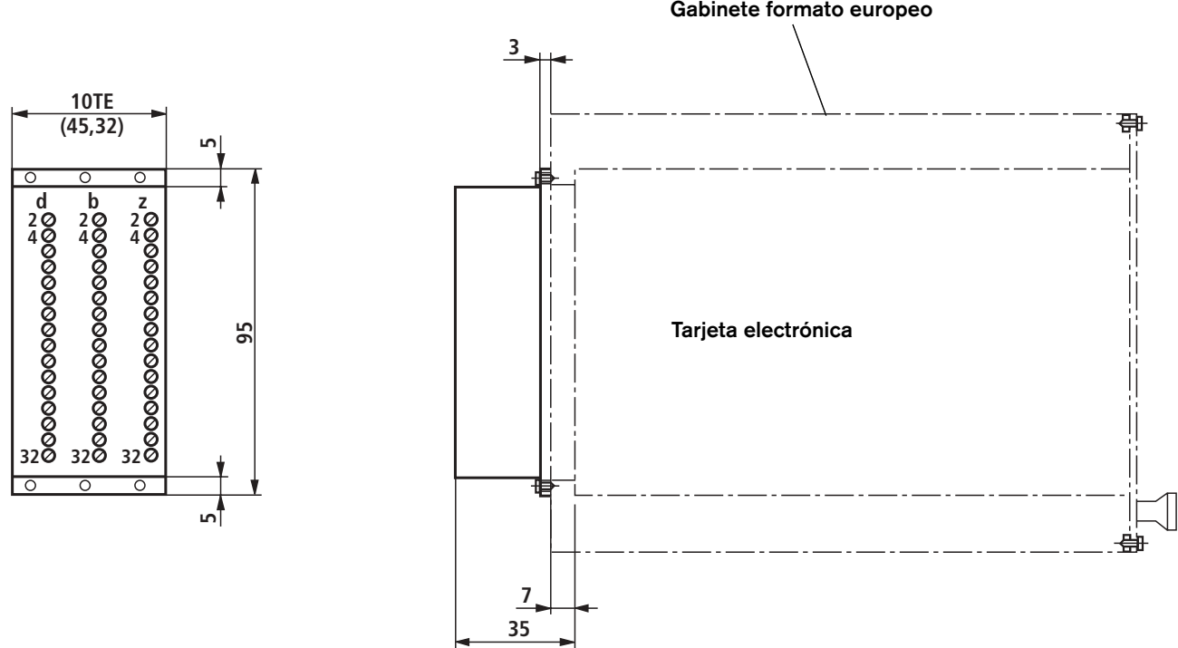
Adaptador, 48 contactos, forma F
