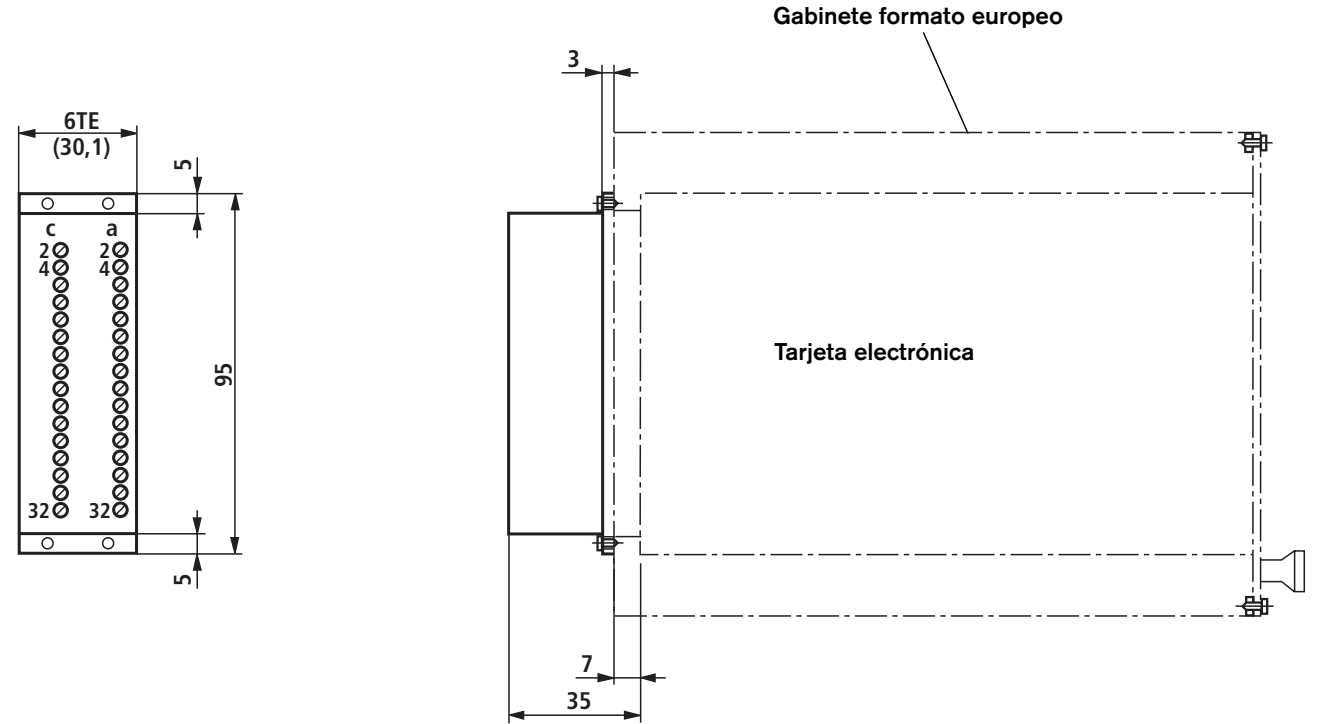
Adaptador, 32 contactos, forma D
